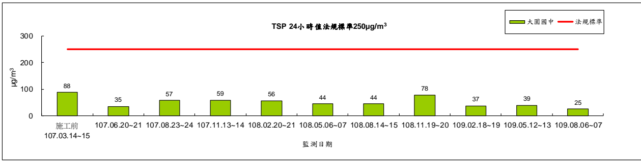
圖 2.1-1 TSP 監測結果趨勢圖
