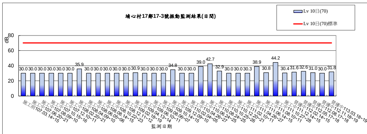
圖 2.2-7 埔心村 17 鄰 17-3 號環境振動監測結果(日間)
