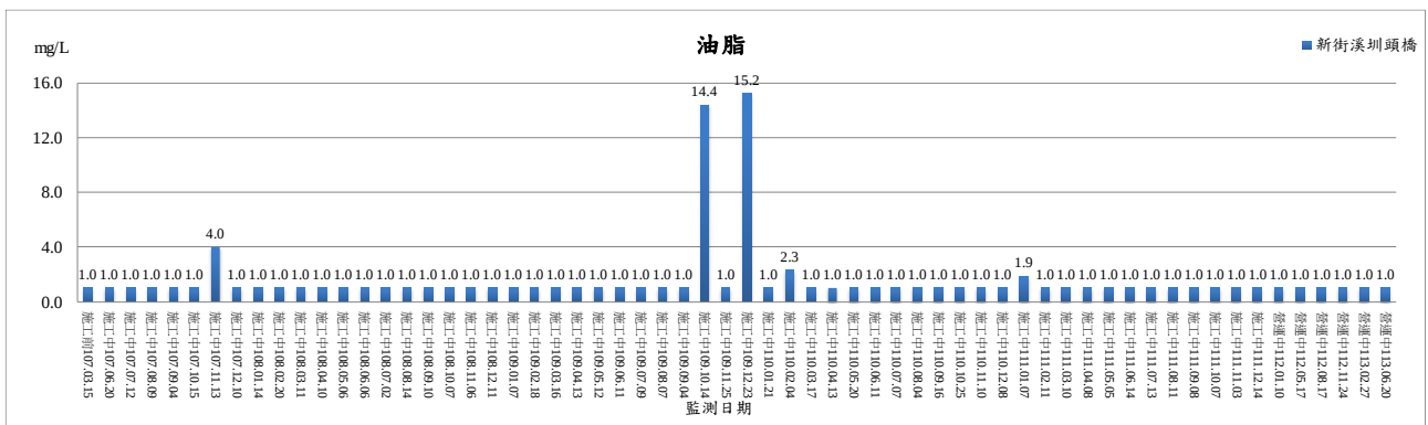
圖 2.3-7 河川水質之油脂監測結果趨勢圖
