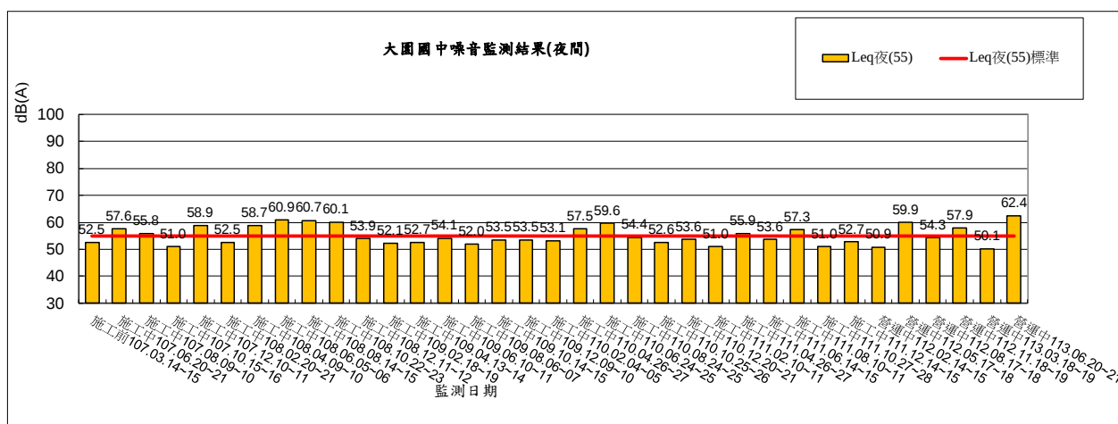
圖 2.2-6 大園國中環境噪音監測結果(夜間)
