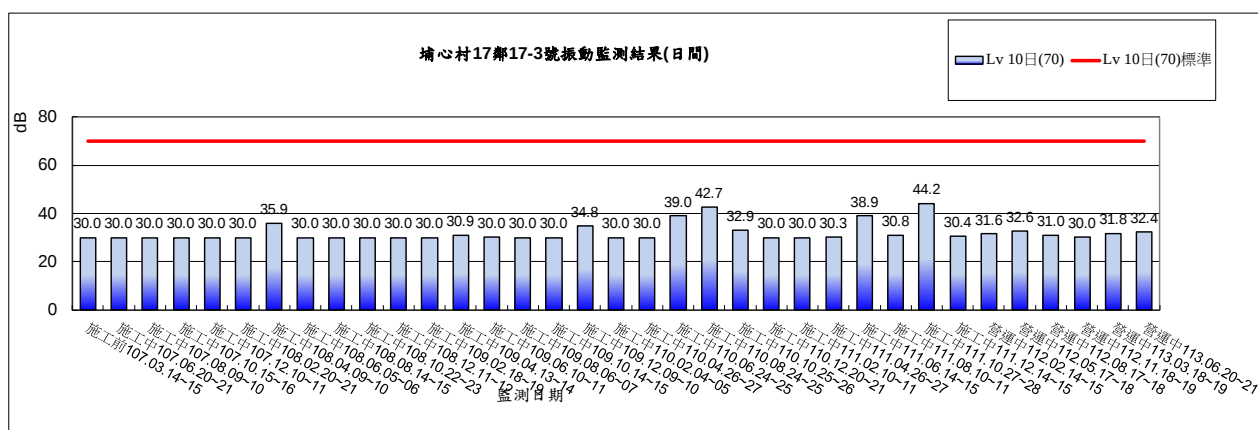
圖 2.2-7 埔心村 17 鄰 17-3 號環境振動監測結果(日間)
