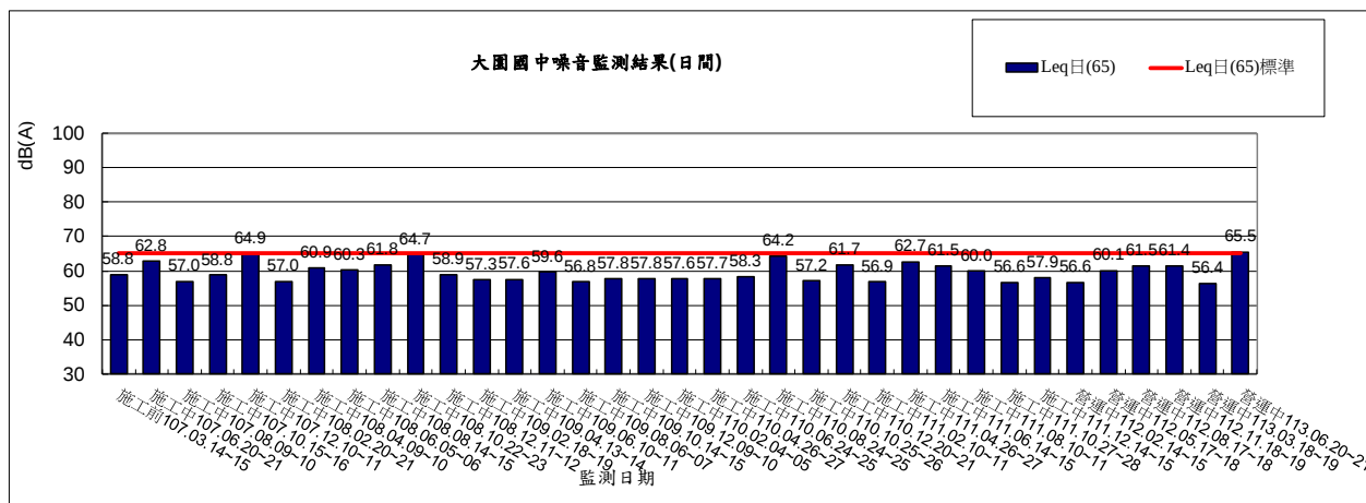
圖 2.2-4 大園國中環境噪音監測結果(日間)
