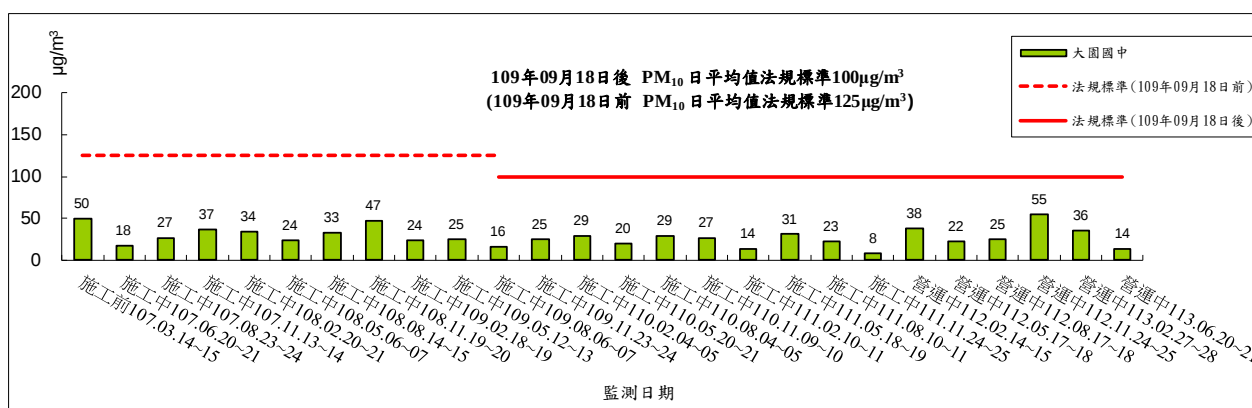
圖 2.1-2 PM 10 監測結果趨勢圖
