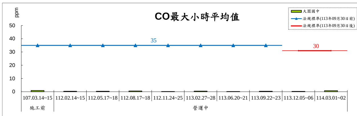
圖 2.1-6 CO 最大小時平均值監測結果趨勢圖
