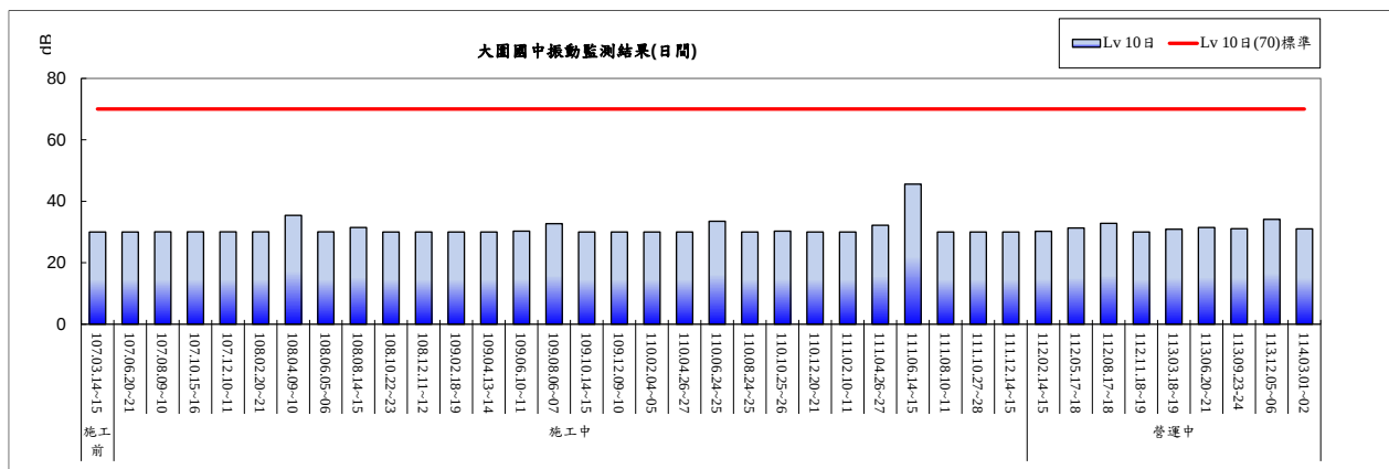
圖 2.2-9 大園國中環境振動監測結果(日間)
