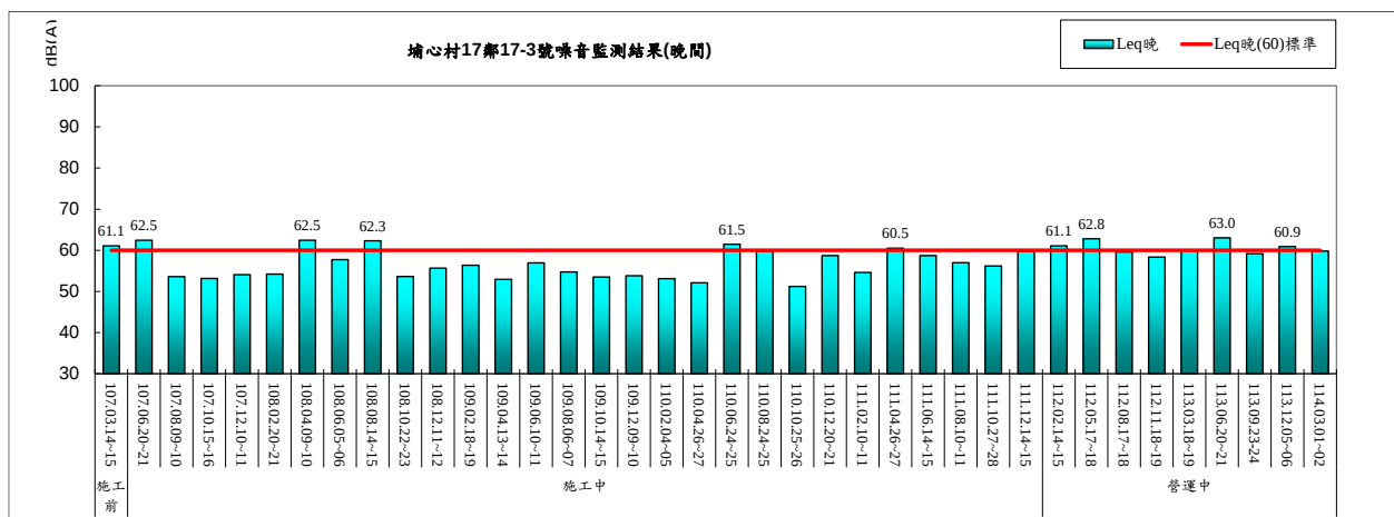
圖 2.2-2 埔心村 17 鄰 17-3 號環境噪音監測結果(晚間)
