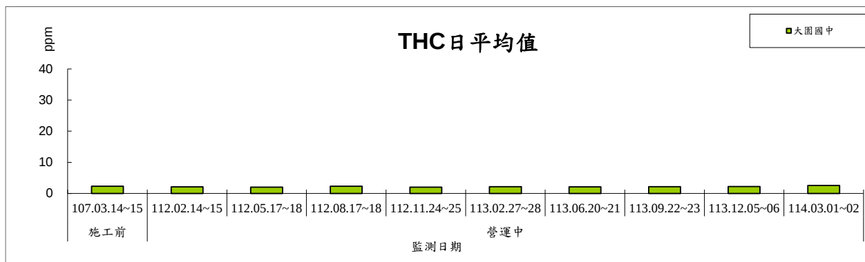
圖 2.1-10 THC 日平均值監測結果趨勢圖
