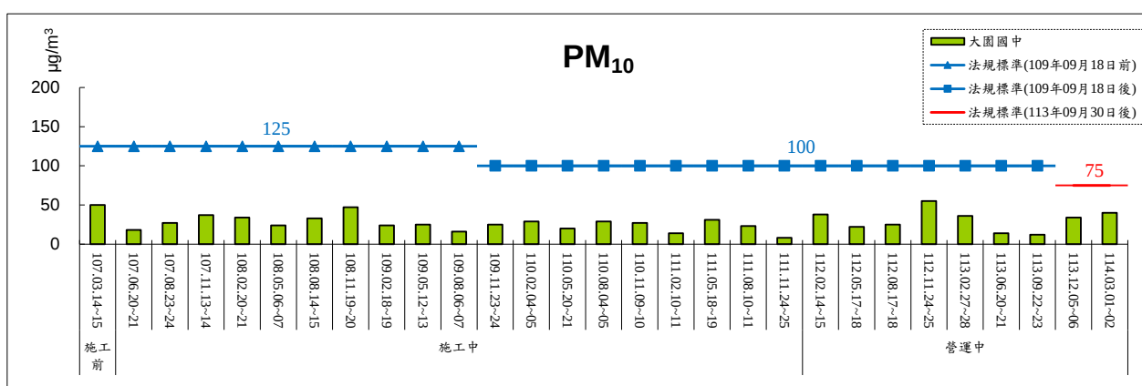
圖 2.1-2 PM 10 監測結果趨勢圖
