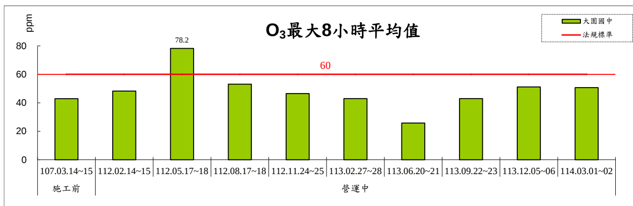
圖 2.1-8 O 3 最大 8 小時平均值監測結果趨勢圖
