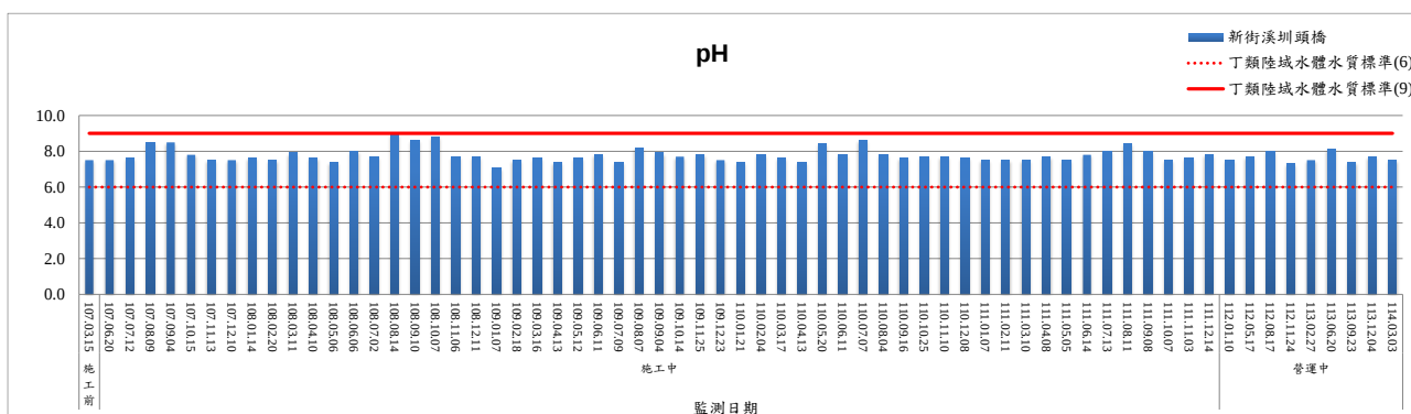
圖 2.3-1 河川水質之 pH 監測結果趨勢圖
