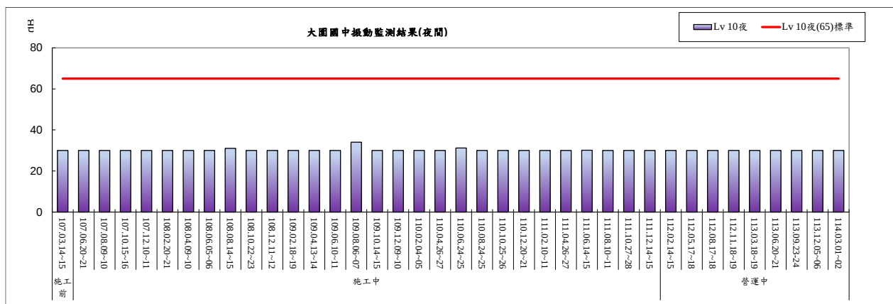
圖 2.2-10 大園國中環境振動監測結果(夜間)
