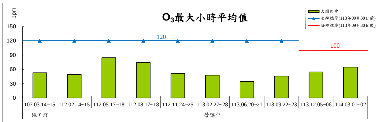
圖 2.1-7 O 3 最大小時平均值監測結果趨勢圖
