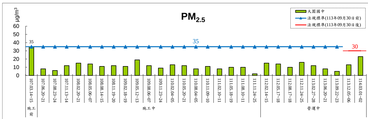
圖 2.1-3 PM 2.5 監測結果趨勢圖
