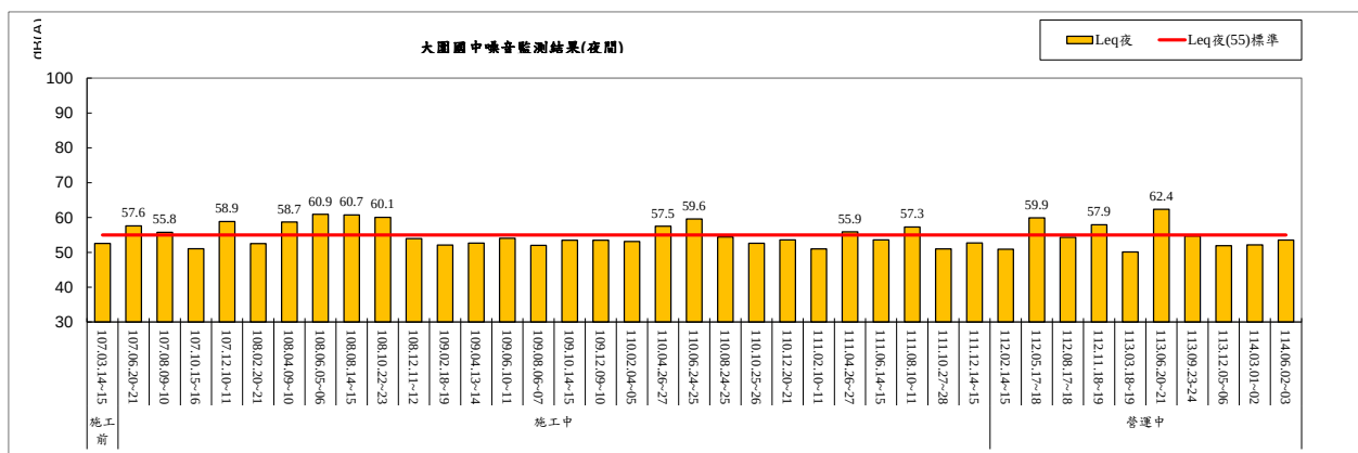
圖 2.2-6 大園國中環境噪音監測結果(夜間)
