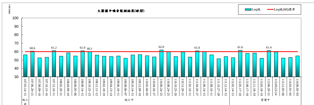
圖 2.2-5 大園國中環境噪音監測結果(晚間)
