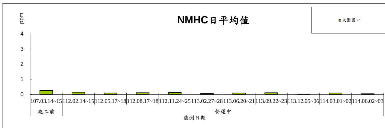
圖 2.1-9 NMHC 日平均值監測結果趨勢圖
