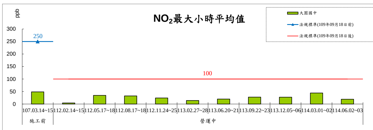
圖 2.1-5 NO 2 最大小時平均值監測結果趨勢圖
