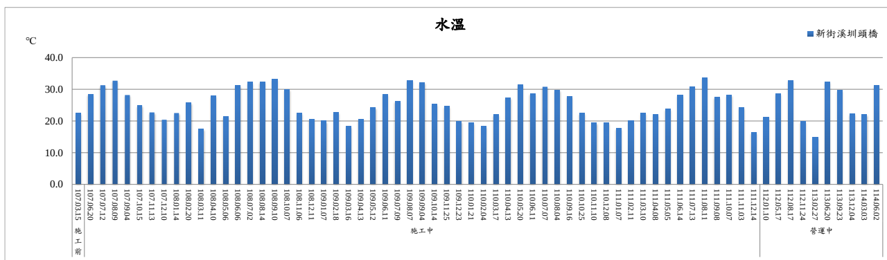
圖 2.3-2 河川水質之水溫監測結果趨勢圖
