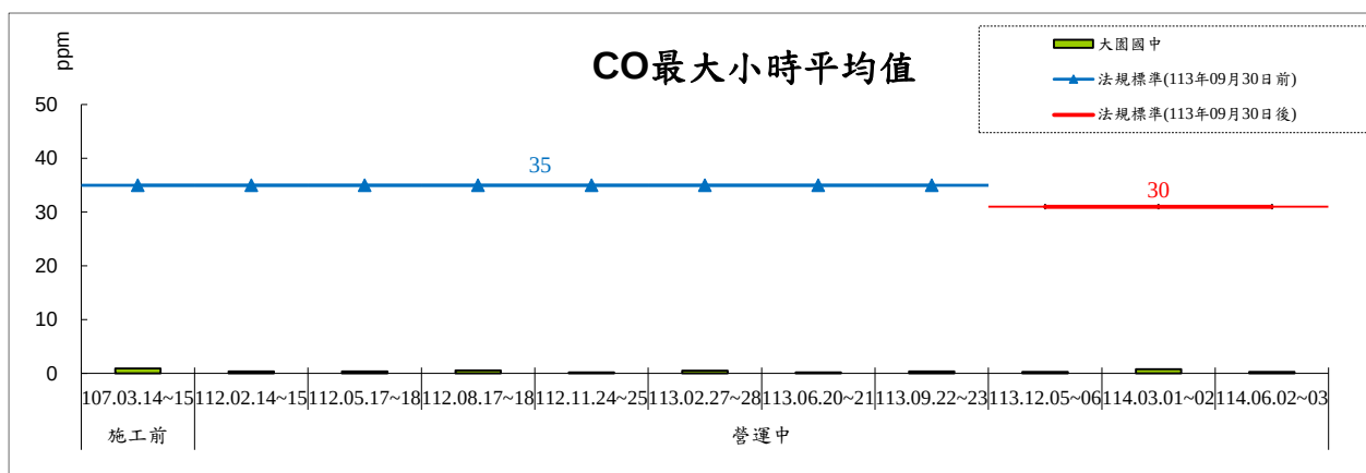
圖 2.1-6 CO 最大小時平均值監測結果趨勢圖
