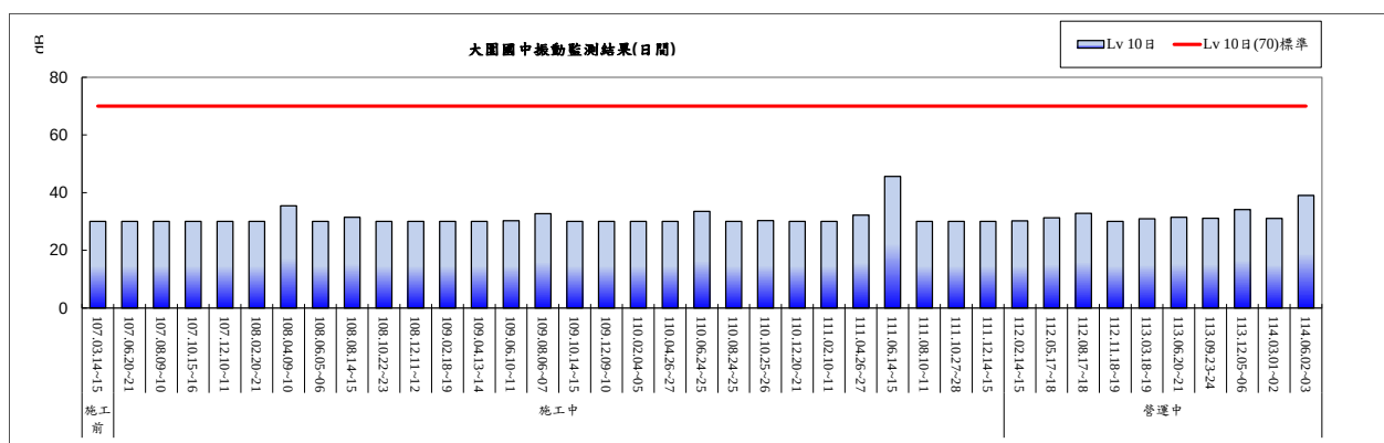
圖 2.2-9 大園國中環境振動監測結果(日間)
