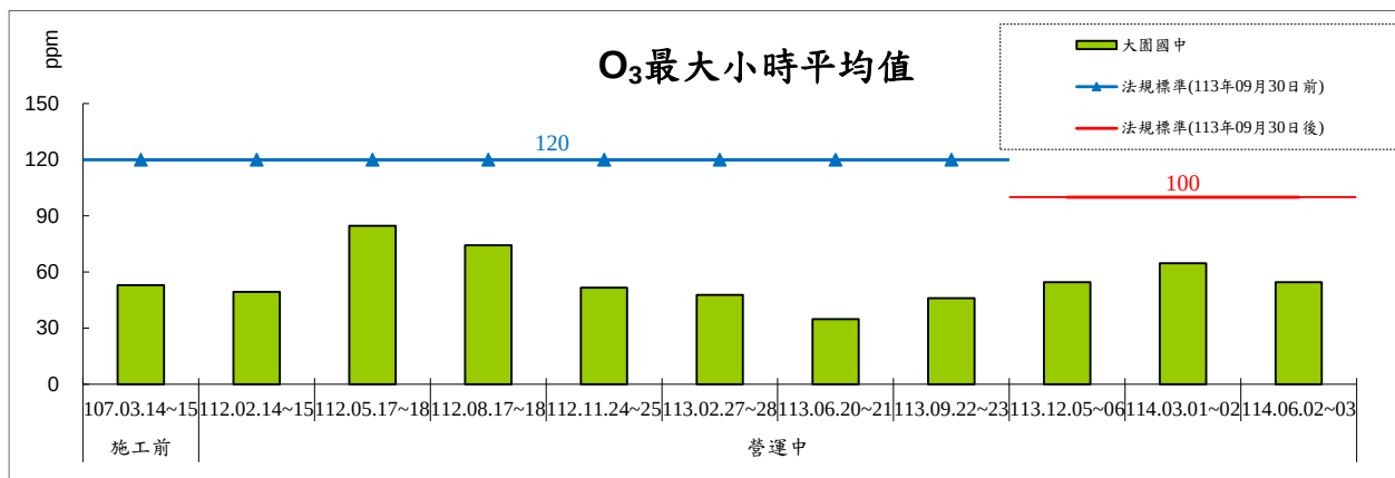
圖 2.1-7 O 3 最大小時平均值監測結果趨勢圖
