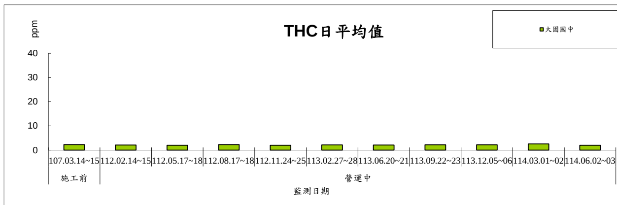
圖 2.1-10 THC 日平均值監測結果趨勢圖
