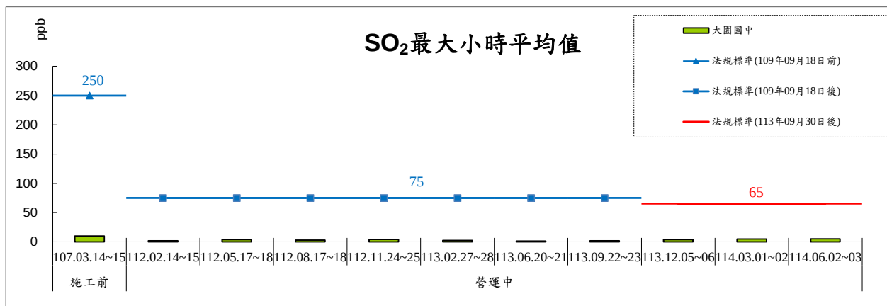
圖 2.1-4 SO 2 最大小時平均值監測結果趨勢圖
