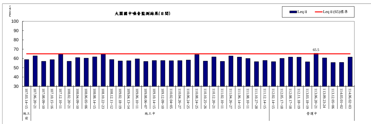
圖 2.2-4 大園國中環境噪音監測結果(日間)
