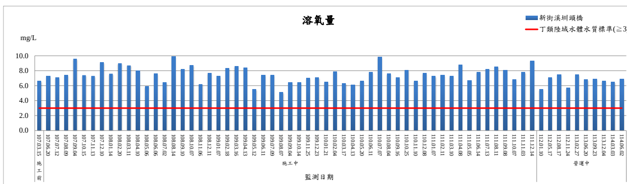
圖 2.3-3 河川水質之溶氧量監測結果趨勢圖
