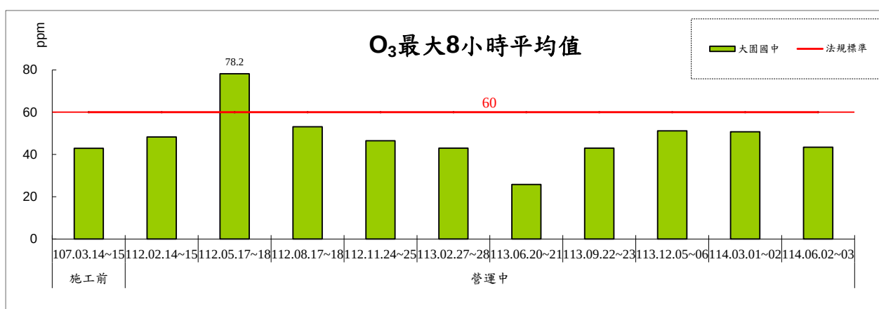
圖 2.1-8 O 3 最大 8 小時平均值監測結果趨勢圖
