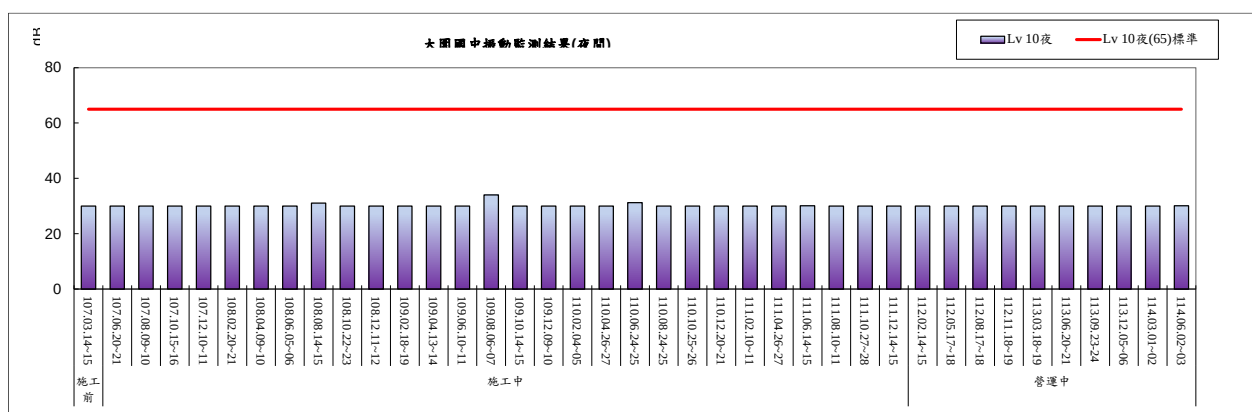
圖 2.2-10 大園國中環境振動監測結果(夜間)
