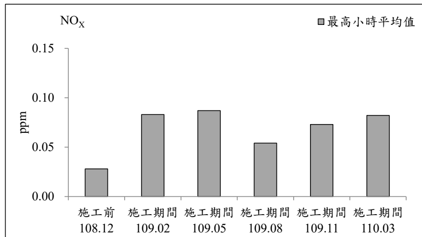
圖 2.1-3 南興路二段 52 巷測站歷次空氣品質監測之各項測值變化圖
