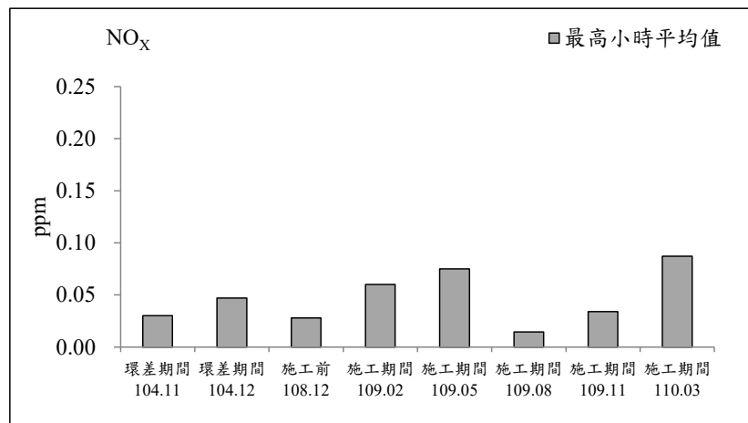
圖 2.1-1 鴻喜鎮社區測站歷次空氣品質監測之各項測值變化圖
