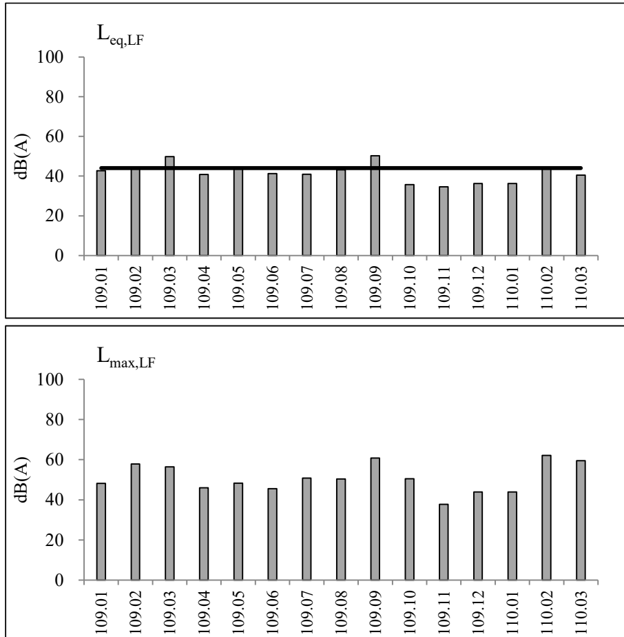
圖 2.6-2 歷次營建低頻噪音監測之各項測值變化圖
