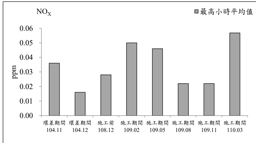
圖 2.1-2 永昌宮測站歷次空氣品質監測之各項測值變化圖
