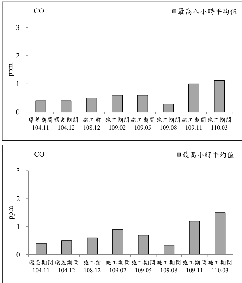
圖 2.1-1 鴻喜鎮社區測站歷次空氣品質監測之各項測值變化圖(續 2)
