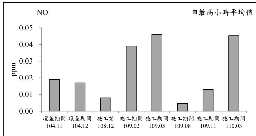
圖 2.1-1 鴻喜鎮社區測站歷次空氣品質監測之各項測值變化圖(續 1)
