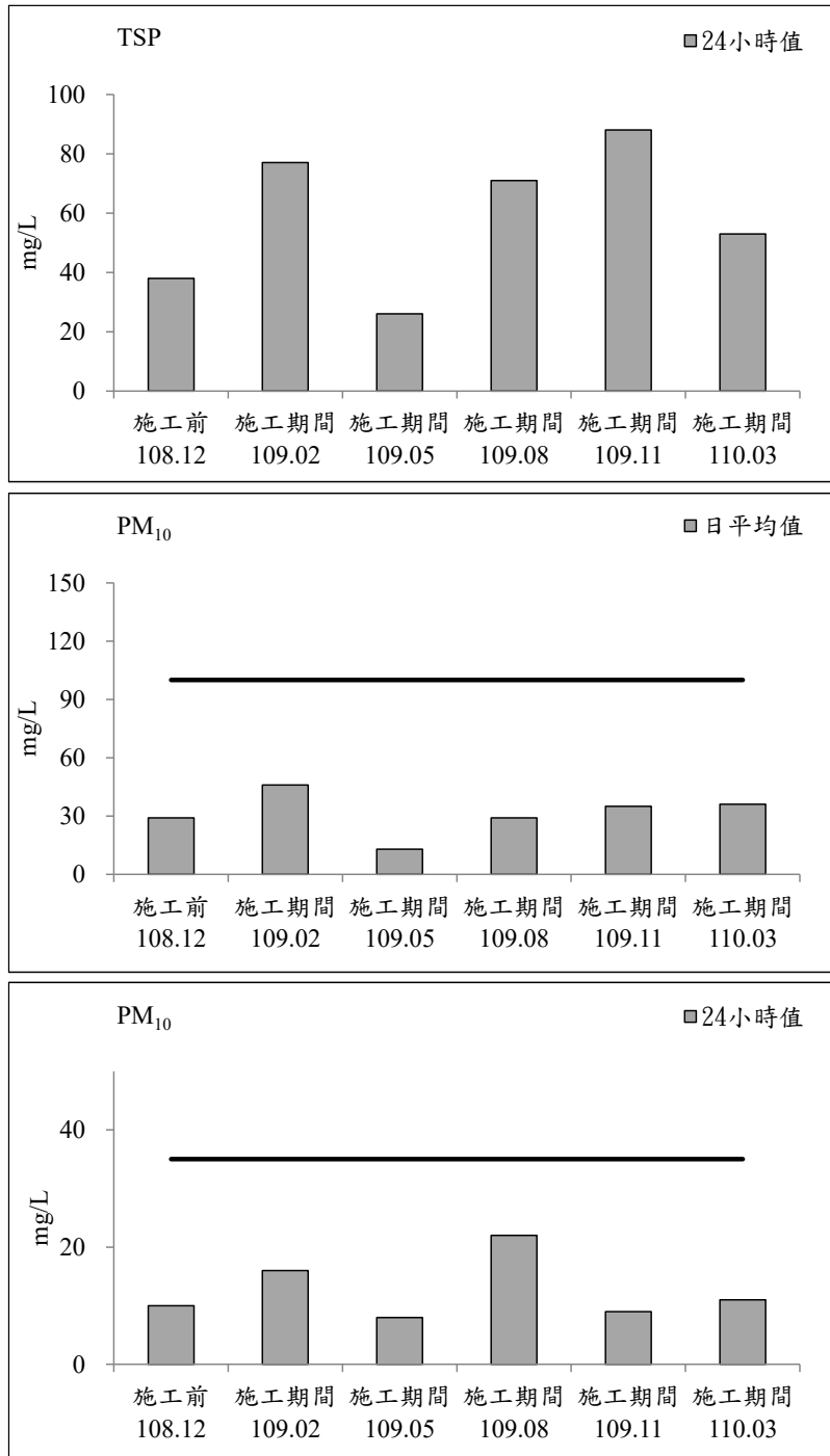
圖 2.1-3 南興路二段 52 巷測站歷次空氣品質監測之各項測值變化圖 (續 3)
