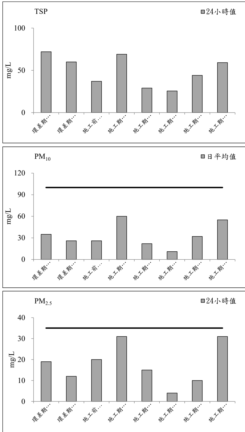
圖 2.1-1 鴻喜鎮社區測站歷次空氣品質監測之各項測值變化圖(續 3)
