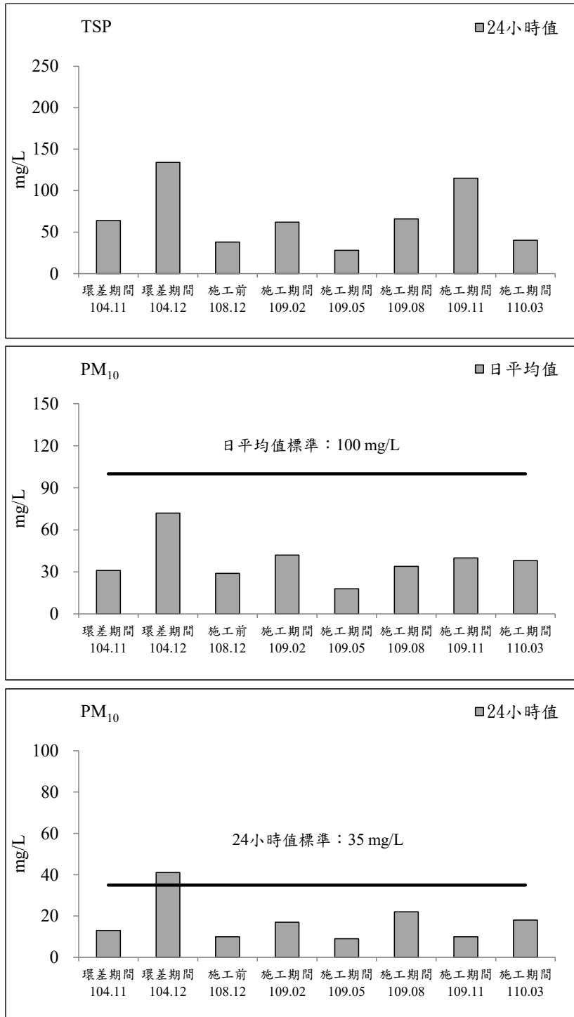
圖 2.1-2 永昌宮測站歷次空氣品質監測之各項測值變化圖(續 3)
