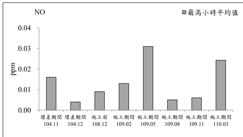
圖 2.1-2 永昌宮測站歷次空氣品質監測之各項測值變化圖(續 1)
