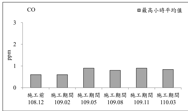
圖 2.1-3 南興路二段 52 巷測站歷次空氣品質監測之各項測值變化圖 (續 2)
