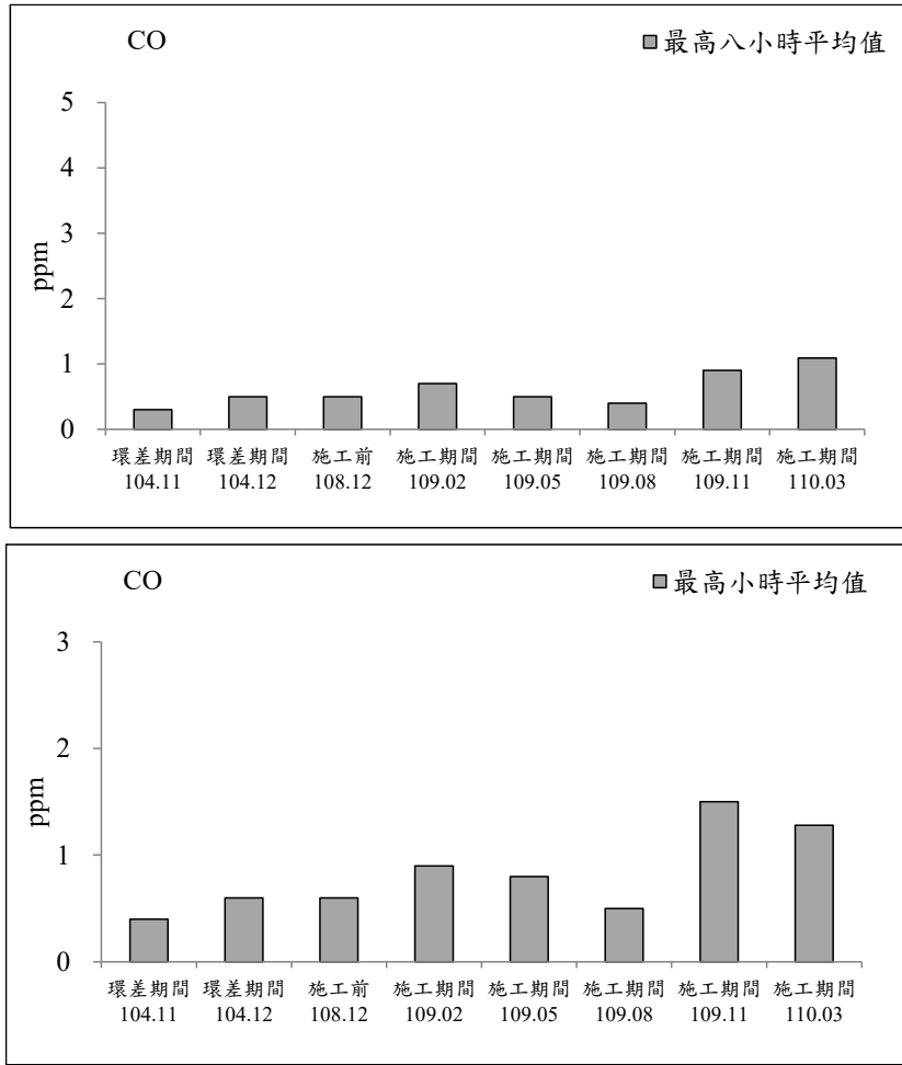
圖 2.1-2 永昌宮測站歷次空氣品質監測之各項測值變化圖(續 2)
