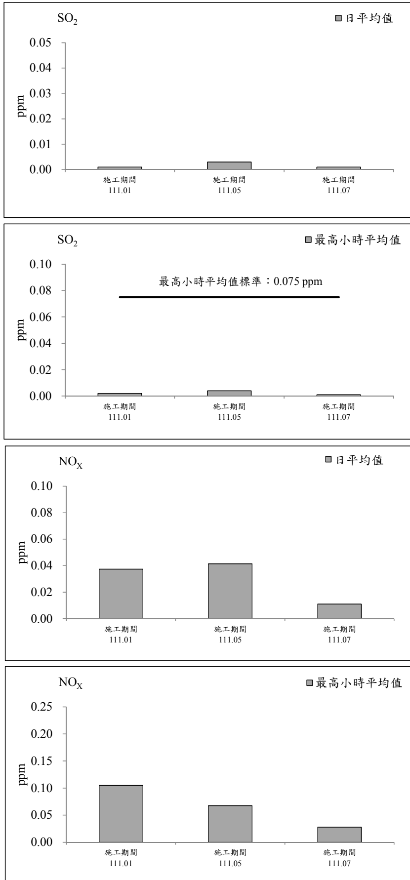
圖 2.1-4 保留戶(南興路二段 230 號民宅)測站歷次空氣品質監測之各項測值變化圖
