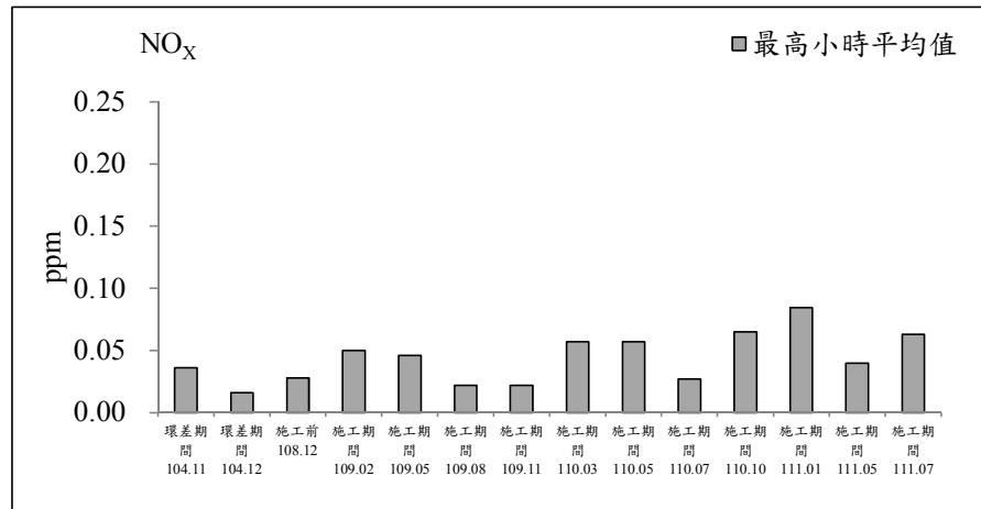
圖 2.1-2 永昌宮測站歷次空氣品質監測之各項測值變化圖
