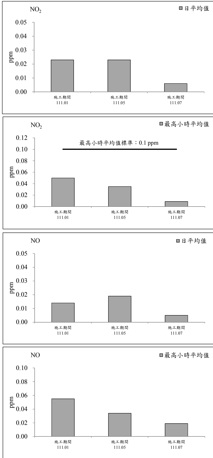
圖 2.1-4 保留戶(南興路二段 230 號民宅)測站歷次空氣品質監測之各項測值變化圖(續 1)
