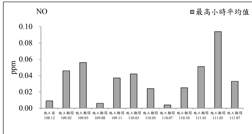
圖 2.1-3 南興路二段 52 巷測站歷次空氣品質監測之各項測值變化圖
