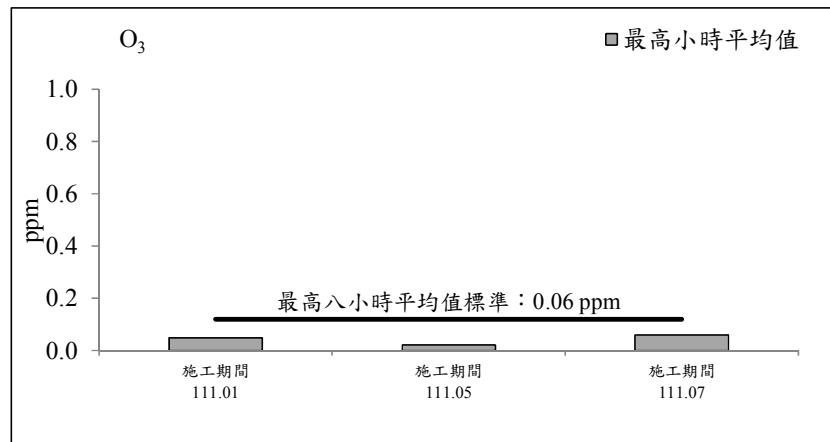
圖 2.1-4 保留戶(南興路二段 230 號民宅)測站歷次空氣品質監測之各項測值變化圖(續 2)
