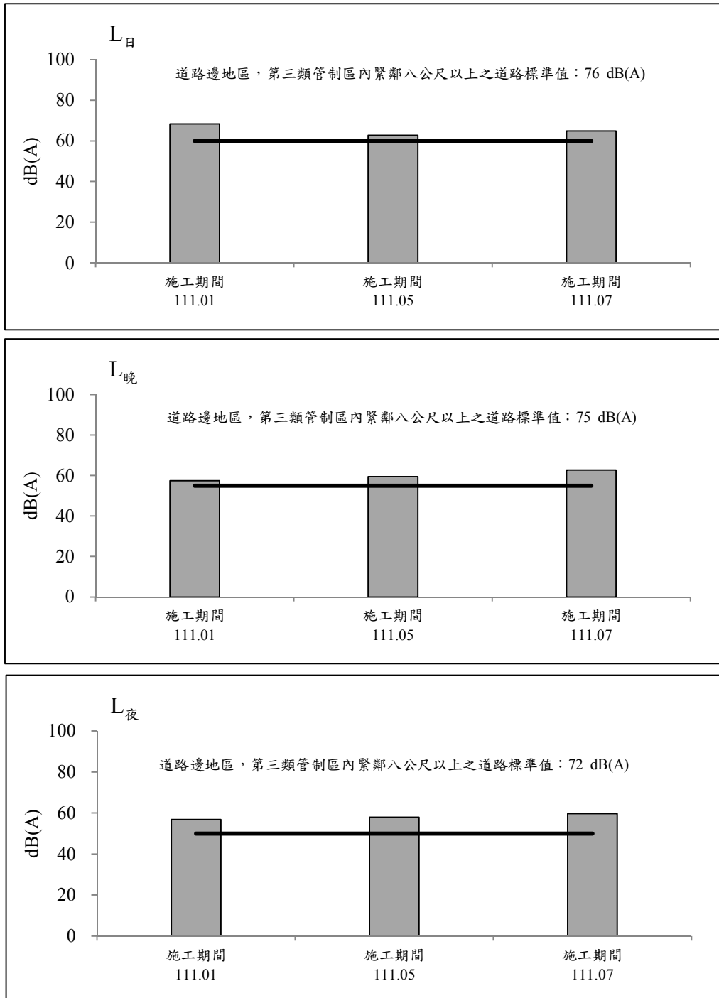
圖 2.2-7 保留戶(南興路二段230號民宅)測站歷次噪音監測之各項測值變化圖(假日)
