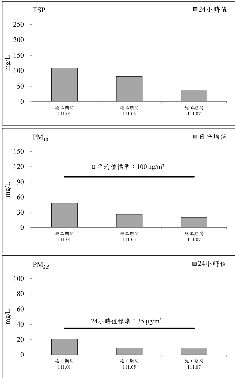
圖 2.1-4 保留戶(南興路二段 230 號民宅)測站歷次空氣品質監測之各項測值變化圖(續 3)
