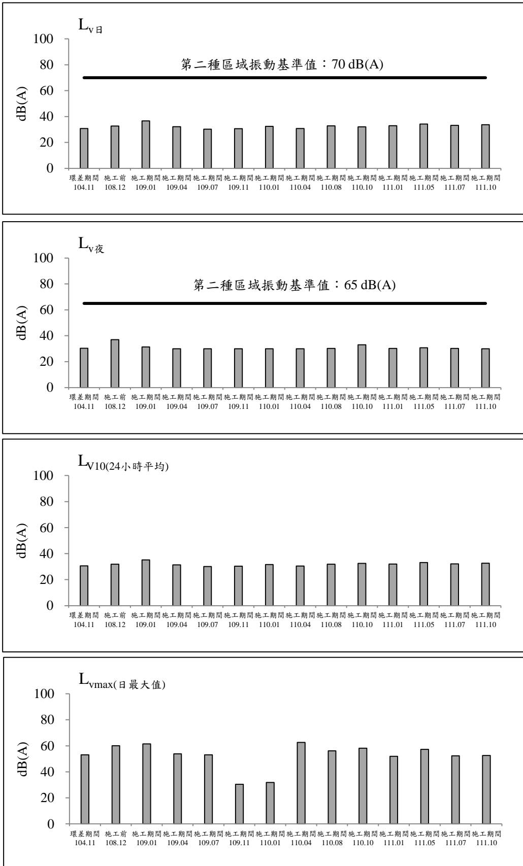
圖 2.2-13 縣112線與縣112甲線交會口測站歷次振動監測之各項測值變化圖(假日)
