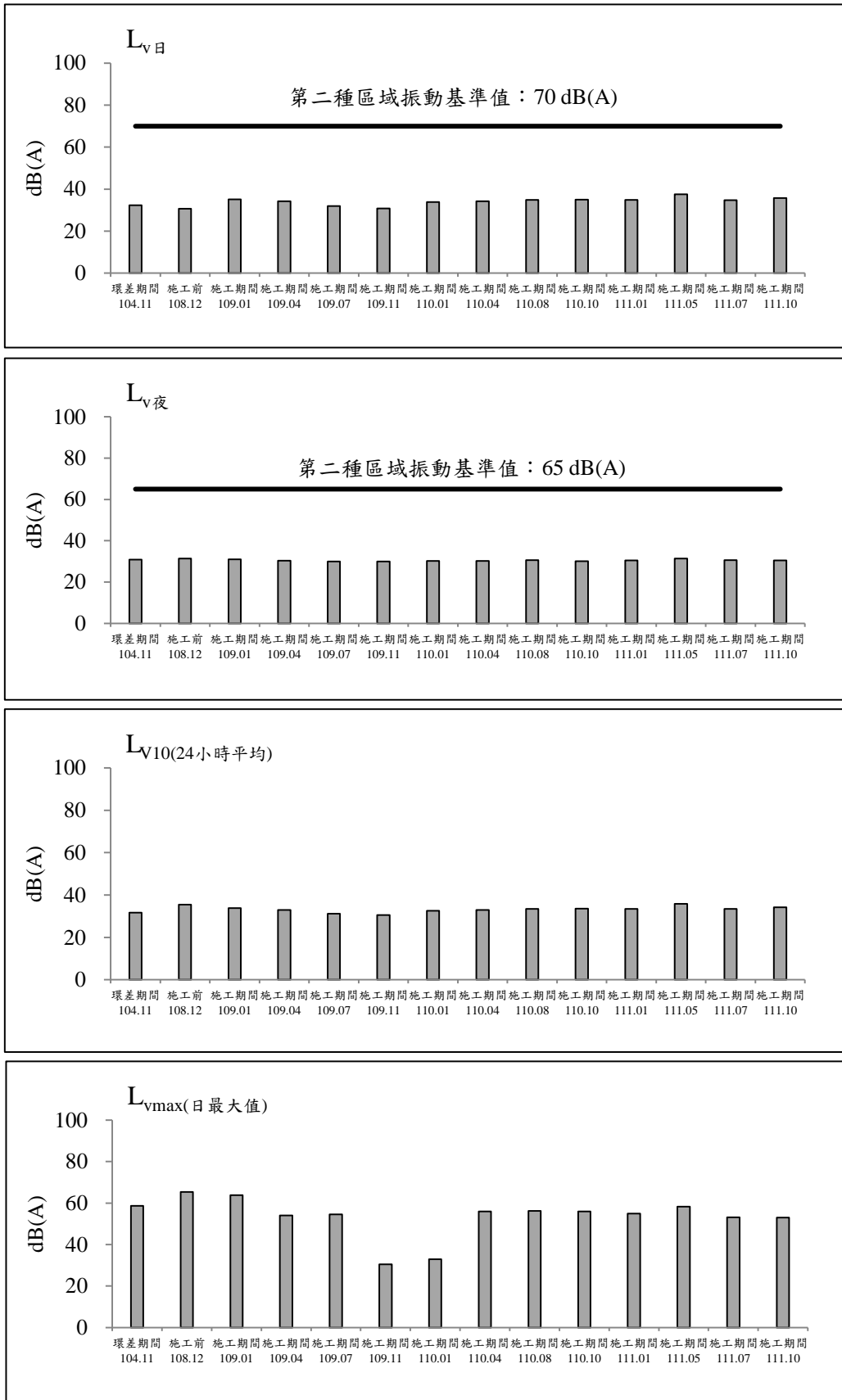
圖 2.2-14 縣112線與縣112甲線交會口測站歷次振動監測之各項測值變化圖(平日)
