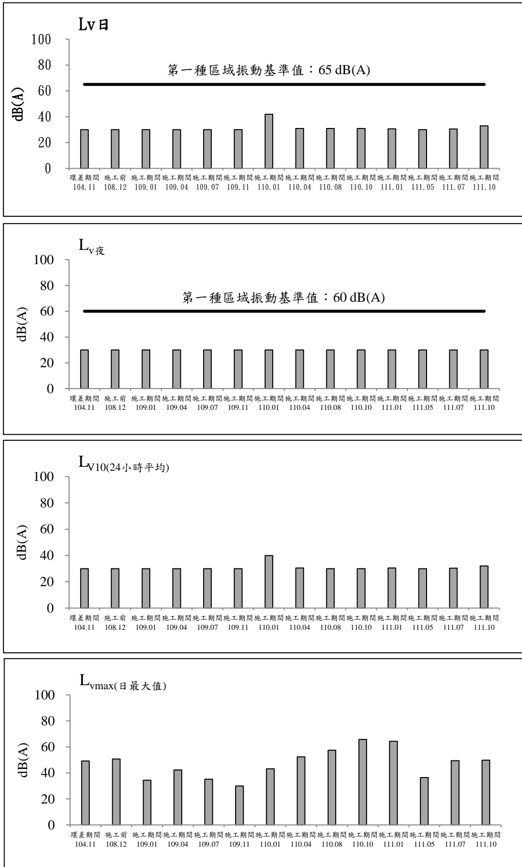
圖 2.2-10 鴻喜鎮社區測站歷次振動監測之各項測值變化圖(平日)
