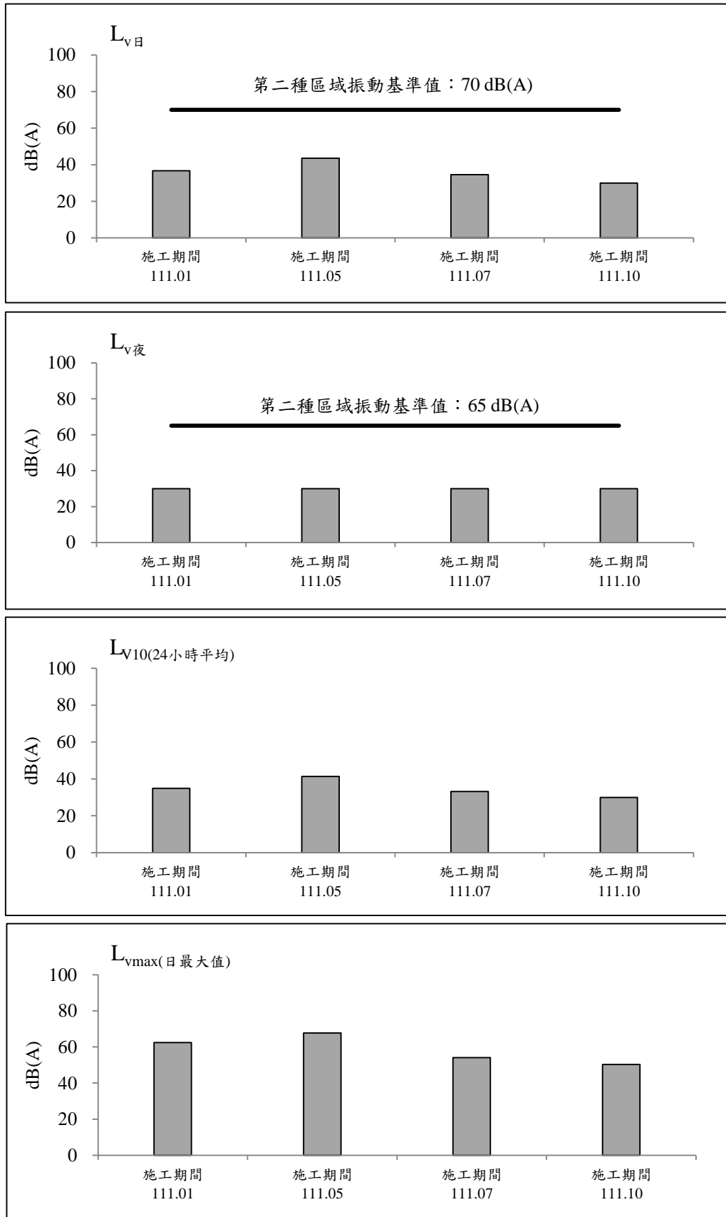
圖 2.2-16 保留戶(南興路二段230號民宅)測站歷次振動監測之各項測值變化圖(平日)
