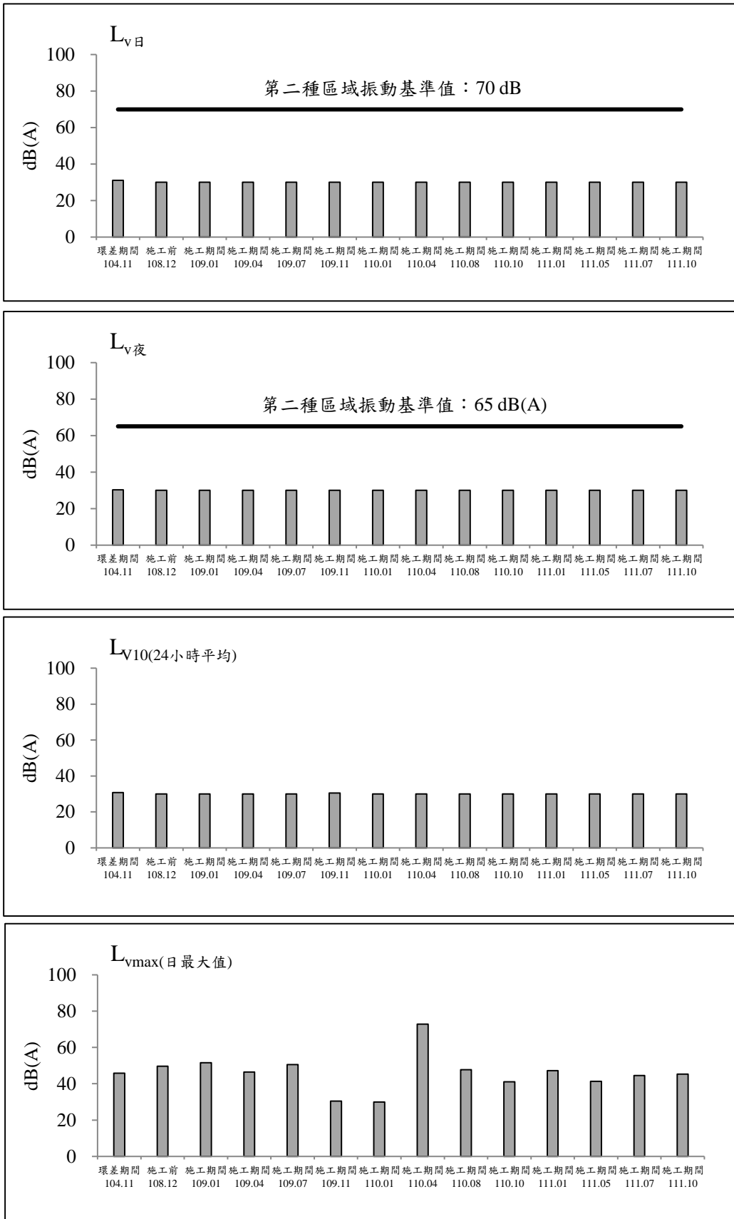
圖 2.2-11 台66線與縣112甲線交會口測站歷次振動監測之各項測值變化圖(假日)
