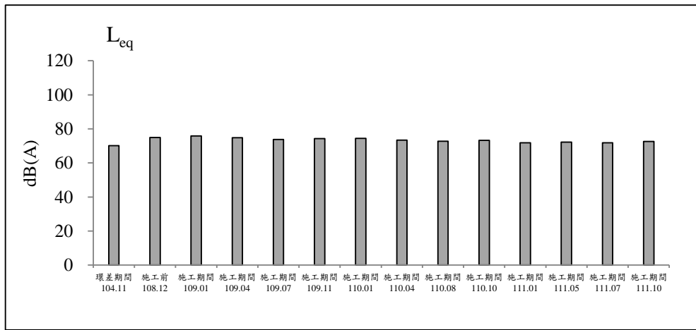
圖 2.2-4 台66線與縣112甲線交會口測站歷次噪音監測之各項測值變化圖(平日)(續)
