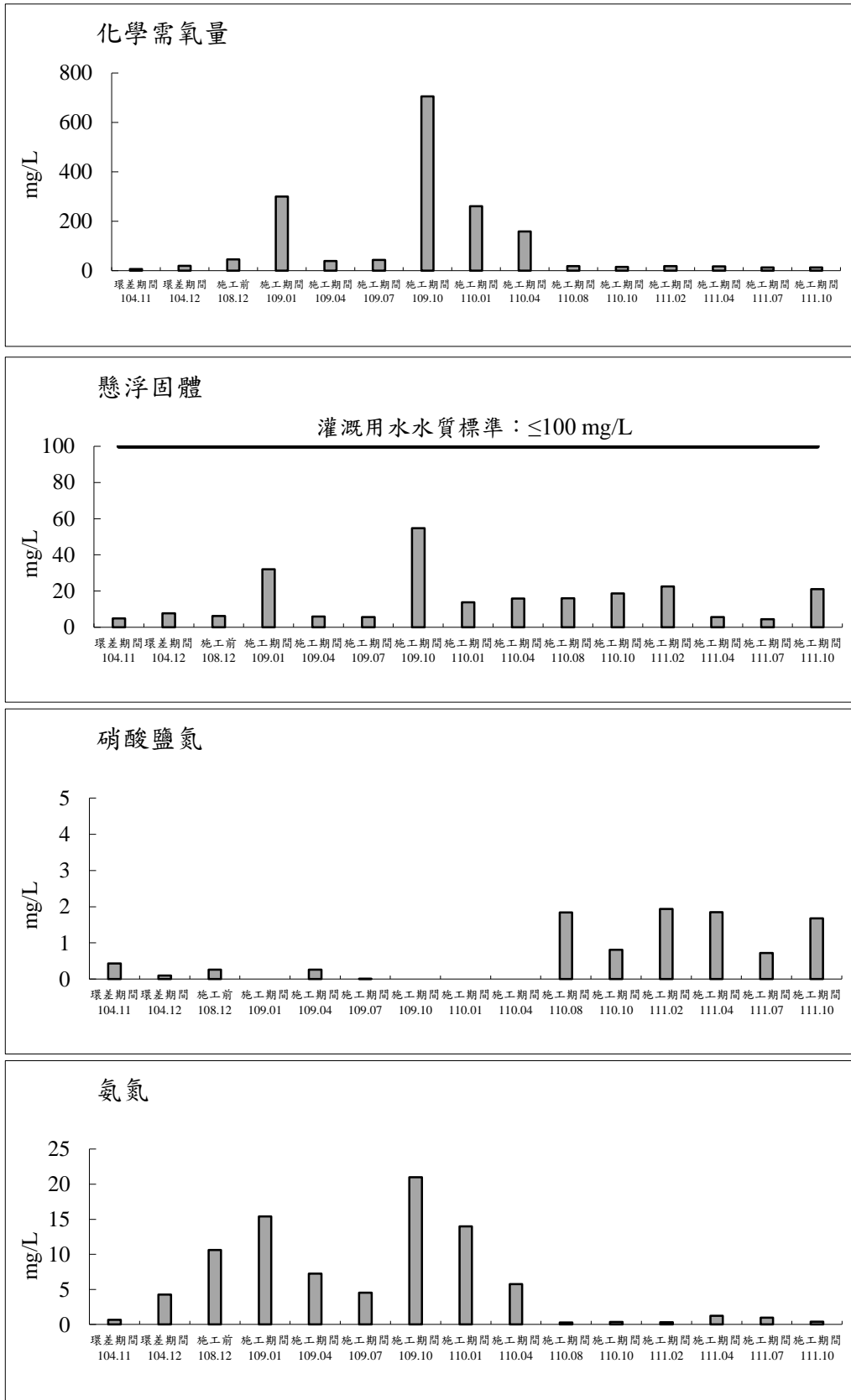
圖 2.3-3 八德分渠(工區下游)測站歷次地面水體水質監測之各項測值變化圖(續 1)
