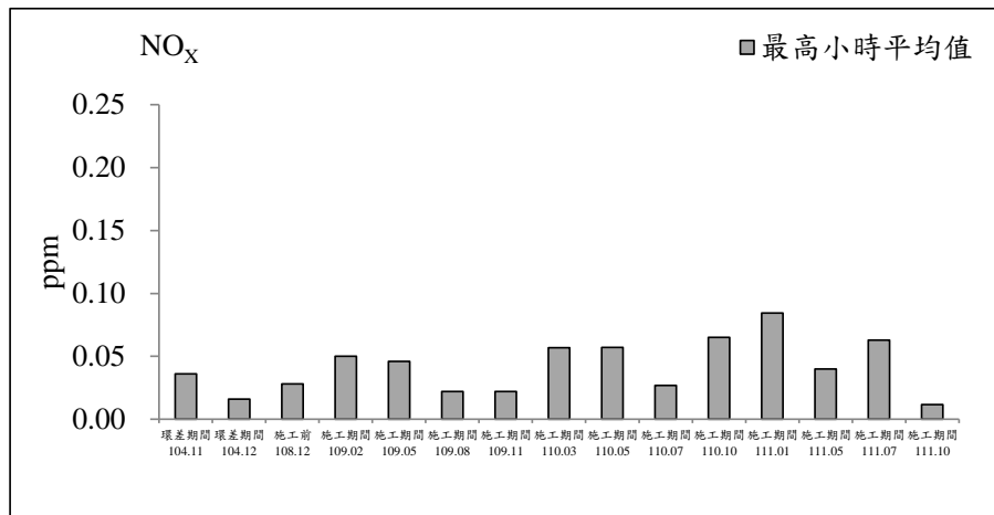
圖 2.1-1 鴻喜鎮社區測站歷次空氣品質監測之各項測值變化圖
