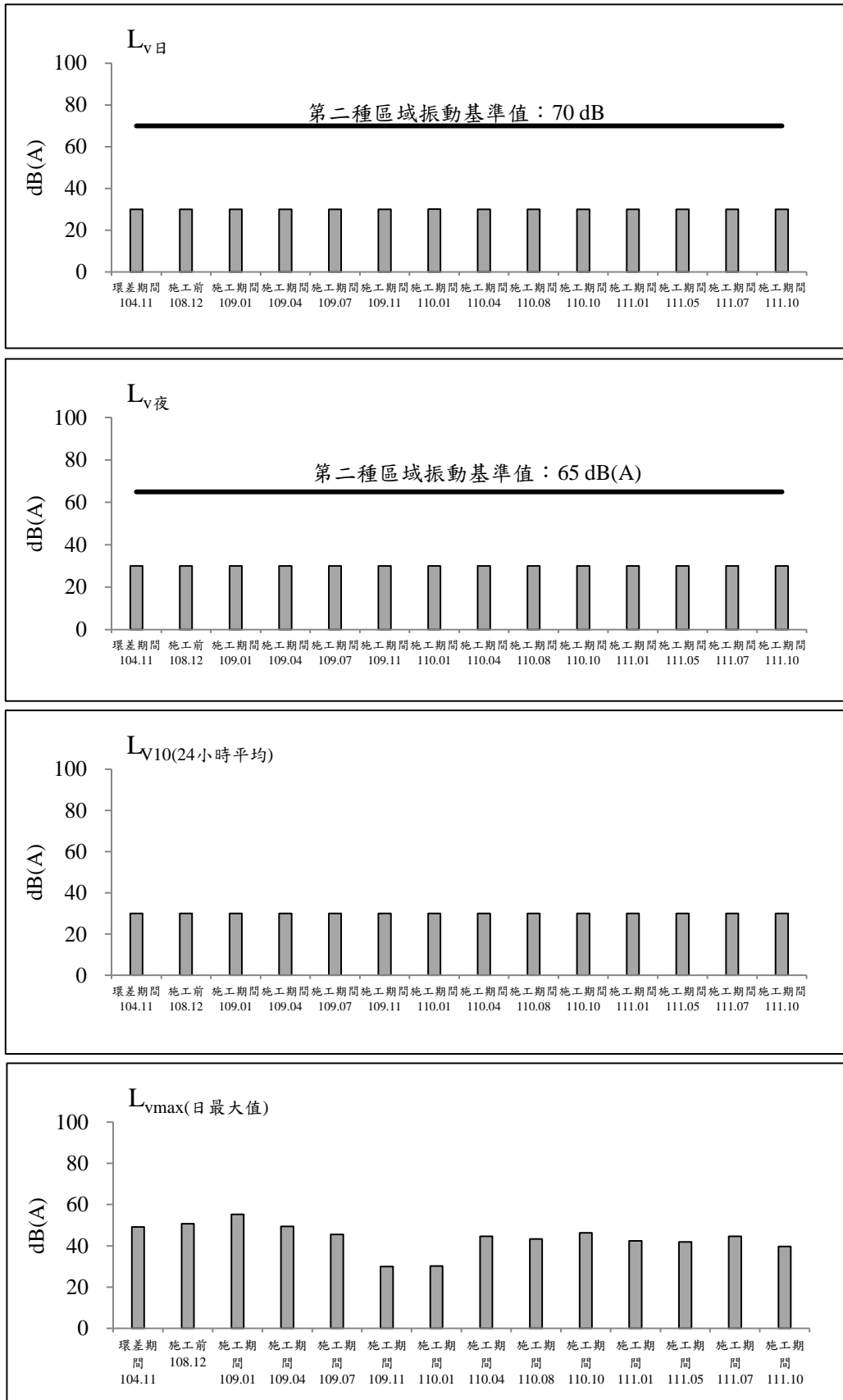
圖 2.2-12 台66線與縣112甲線交會口測站歷次振動監測之各項測值變化圖(平日)
