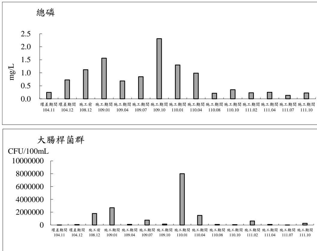
圖 2.3-3 八德分渠(工區下游)測站歷次地面水體水質監測之各項測值變化圖(續 2)
