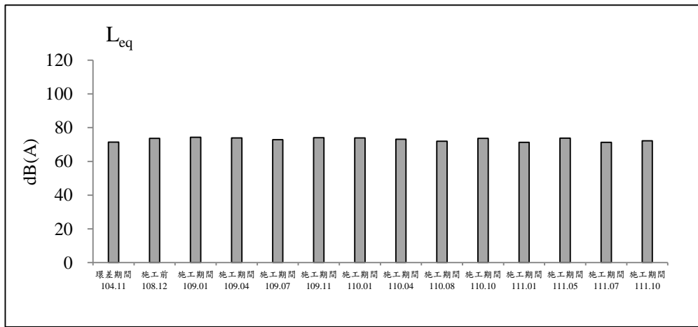
圖 2.2-3 台66線與縣112甲線交會口測站歷次噪音監測之各項測值變化圖(假日)(續)
