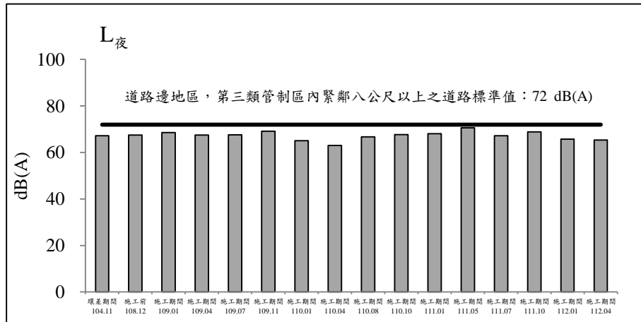
圖 2.2-5 縣112線與縣112甲線交會口測站歷次噪音監測之各項測值變化圖(假日)
