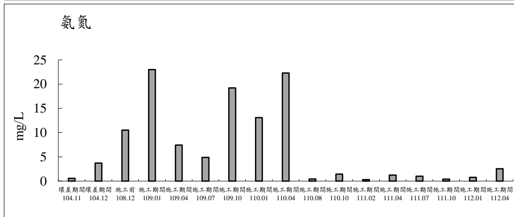
圖 2.3-2 八德分渠(工區上游)測站歷次地面水體水質監測之各項測值變化圖(續 1)
