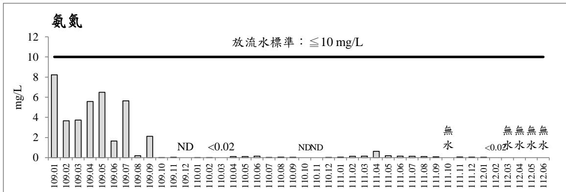
圖 2.7-1 歷次第一工區放流水監測之各項測值變化圖(續)
