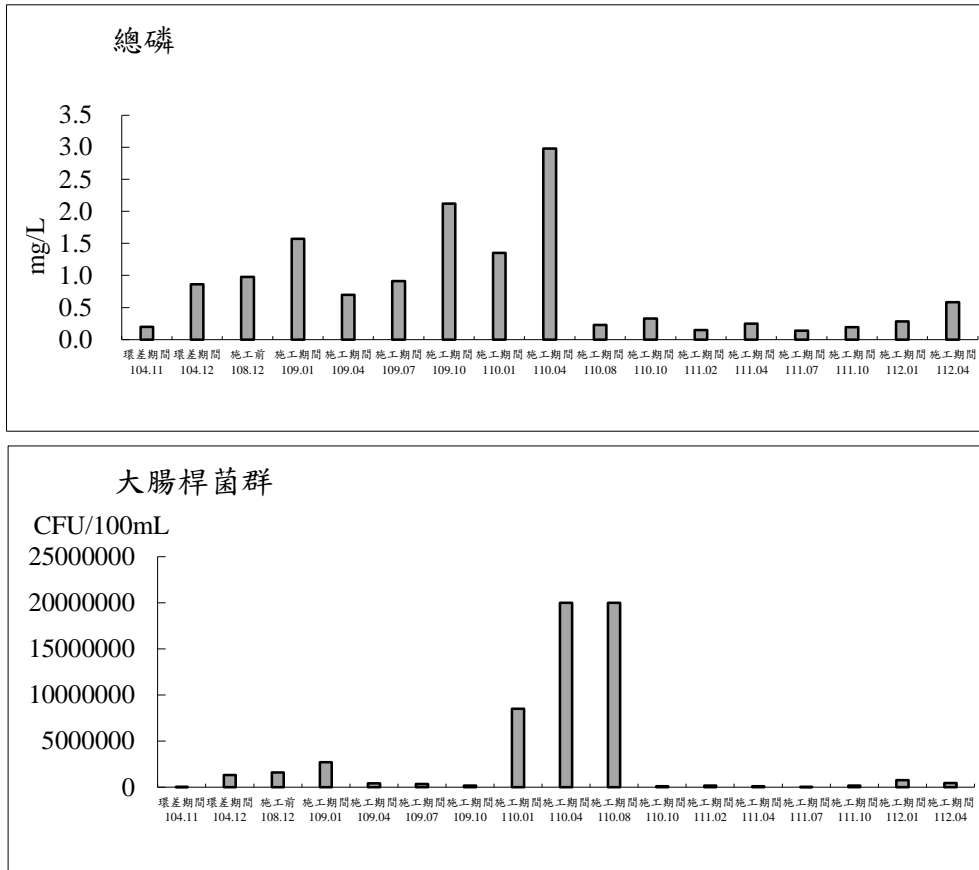
圖 2.3-2 八德分渠(工區上游)測站歷次地面水體水質監測之各項測值變化圖(續 2)
