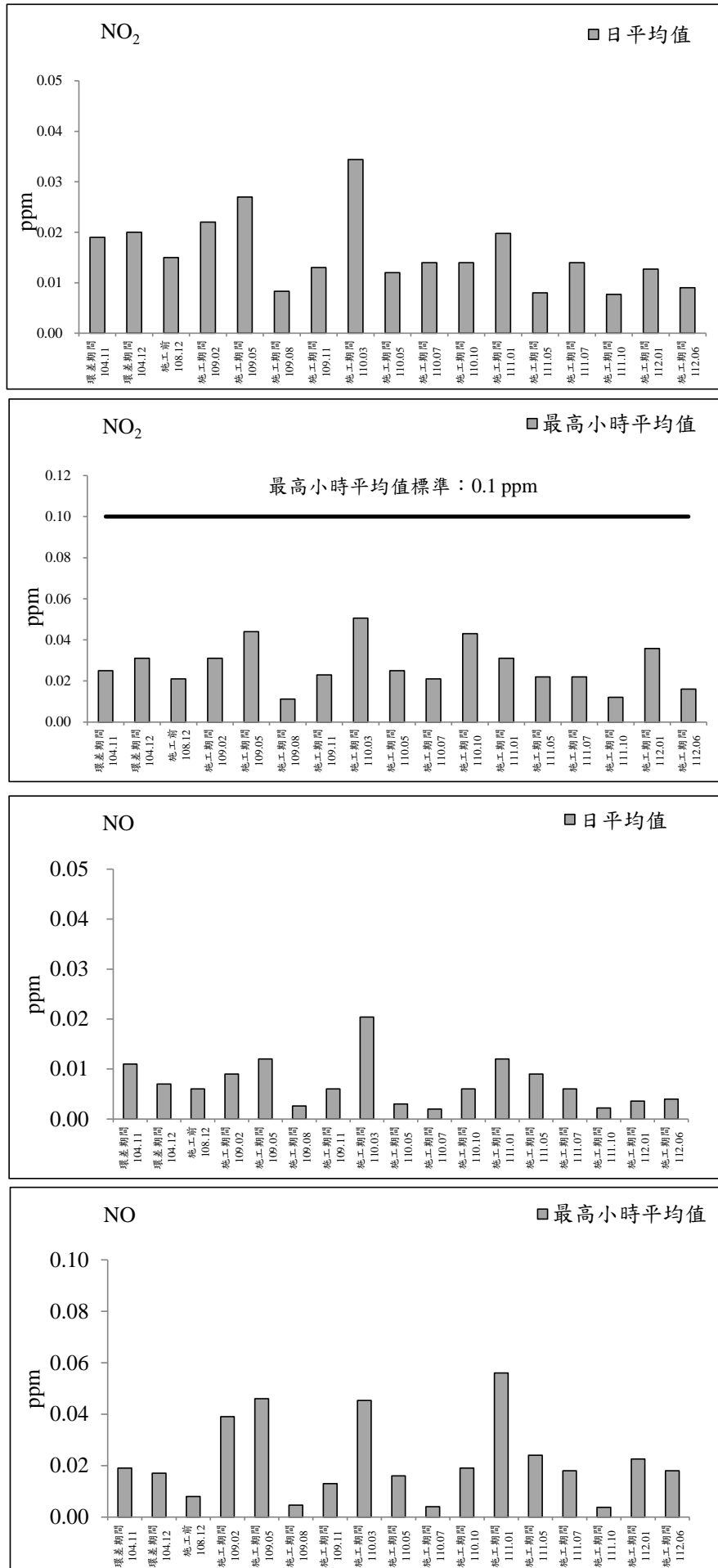
圖 2.1-1 鴻喜鎮社區測站歷次空氣品質監測之各項測值變化圖(續 1)
