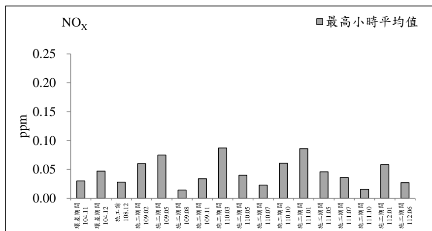
圖 2.1-1 鴻喜鎮社區測站歷次空氣品質監測之各項測值變化圖
