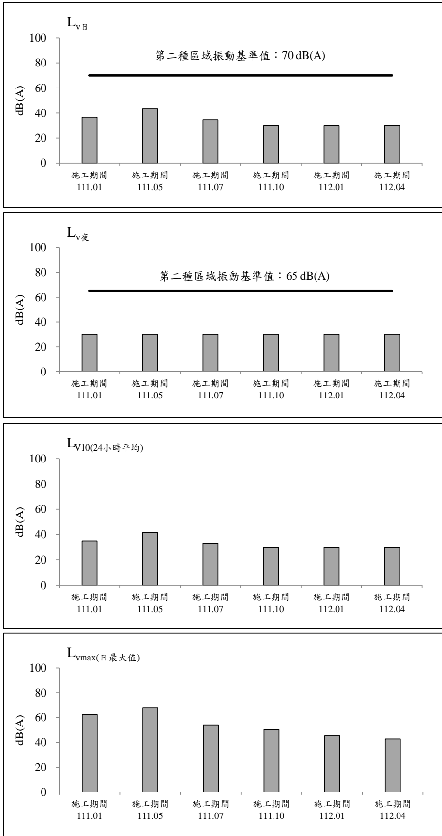
圖 2.2-16 保留戶(南興路二段230號民宅)測站歷次振動監測之各項測值變化圖(平日)
