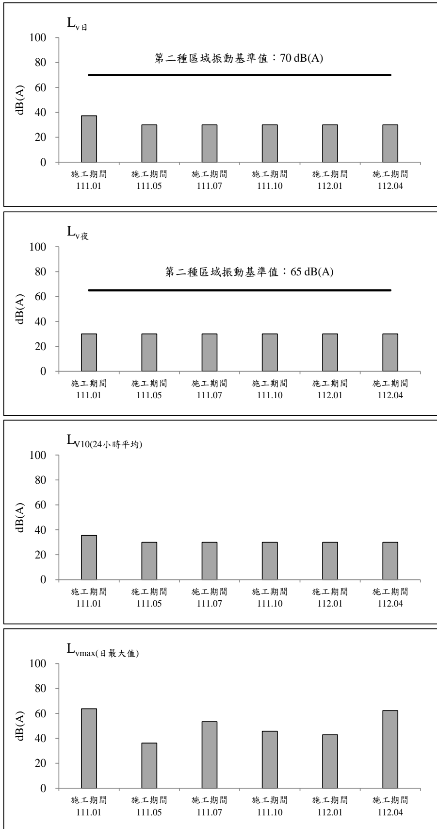
圖 2.2-15 保留戶(南興路二段230號民宅)測站歷次振動監測之各項測值變化圖(假日)
