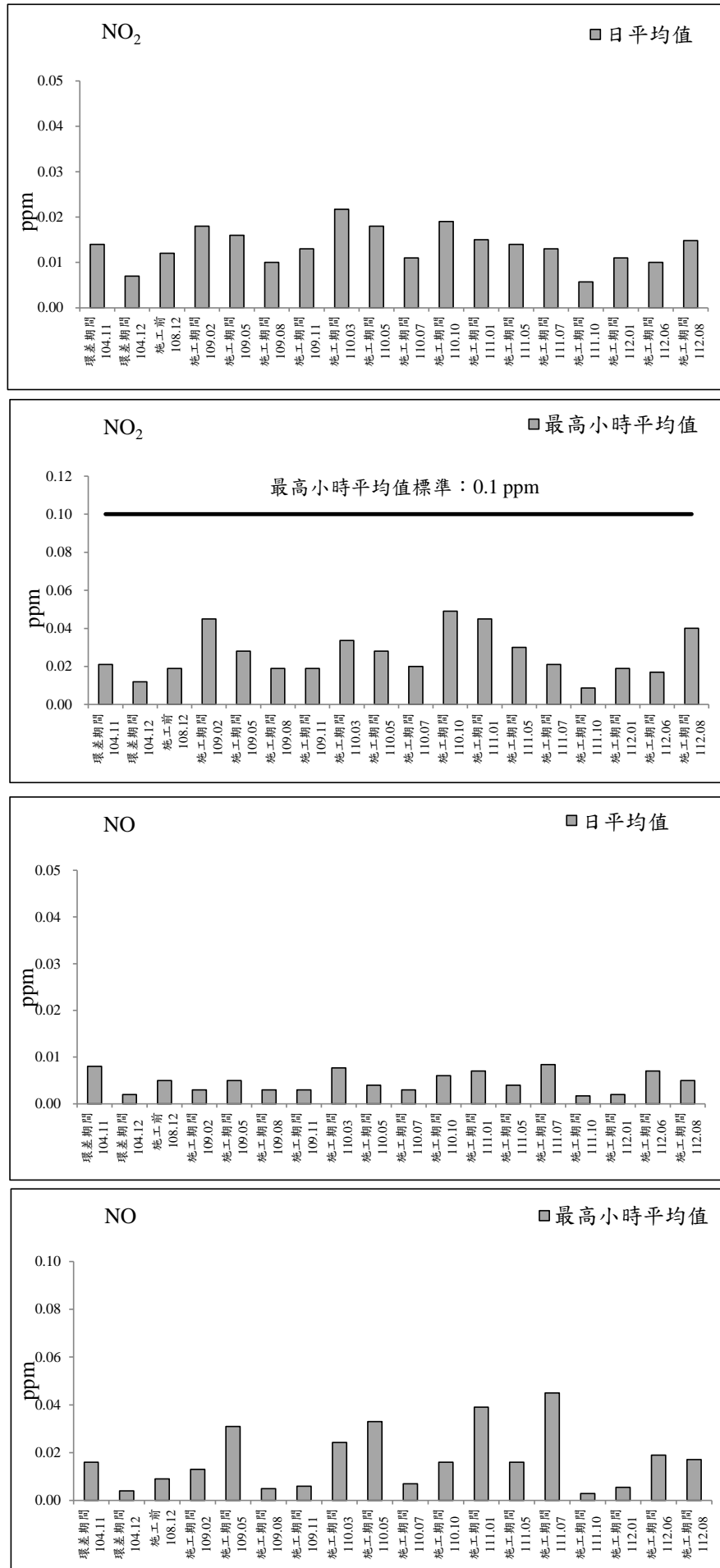
圖 2.1-2 永昌宮測站歷次空氣品質監測之各項測值變化圖(續 1)
