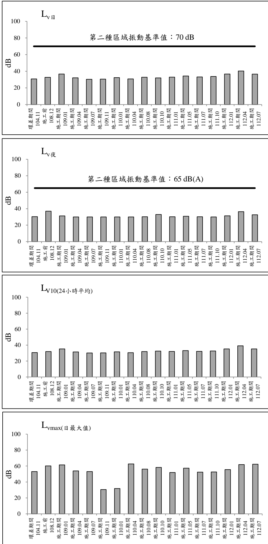
圖 2.2-13 縣112線與縣112甲線交會口測站歷次振動監測之各項測值變化圖(假日)
