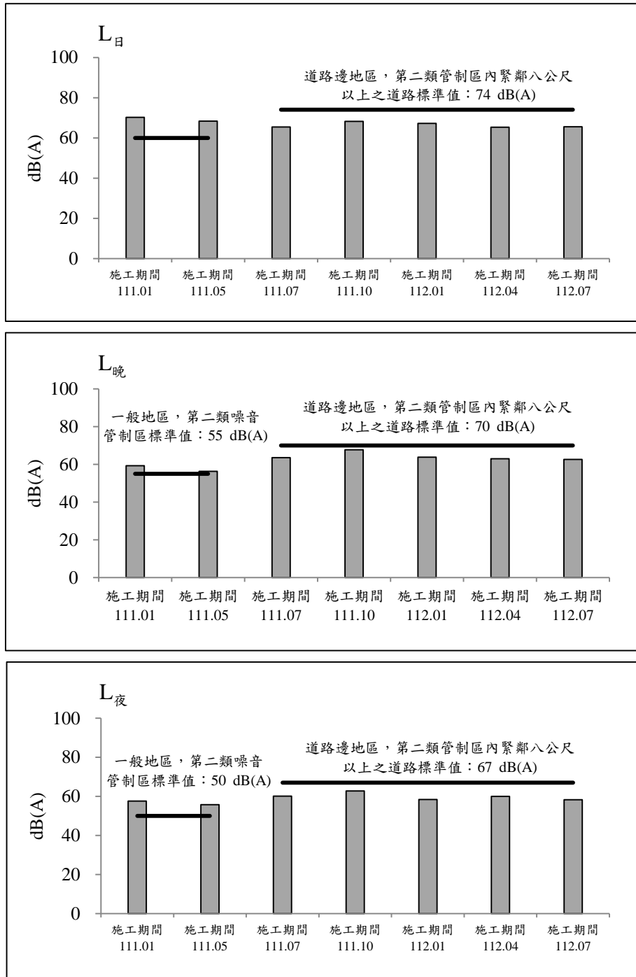
圖 2.2-8 保留戶(南興路二段230號民宅)測站歷次噪音監測之各項測值變化圖(平日)
