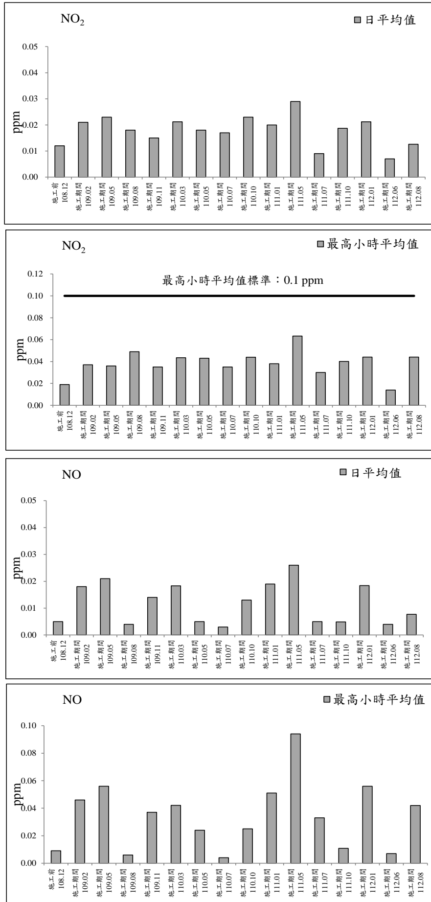
圖 2.1-3 南興路二段 52 巷測站歷次空氣品質監測之各項測值變化圖
