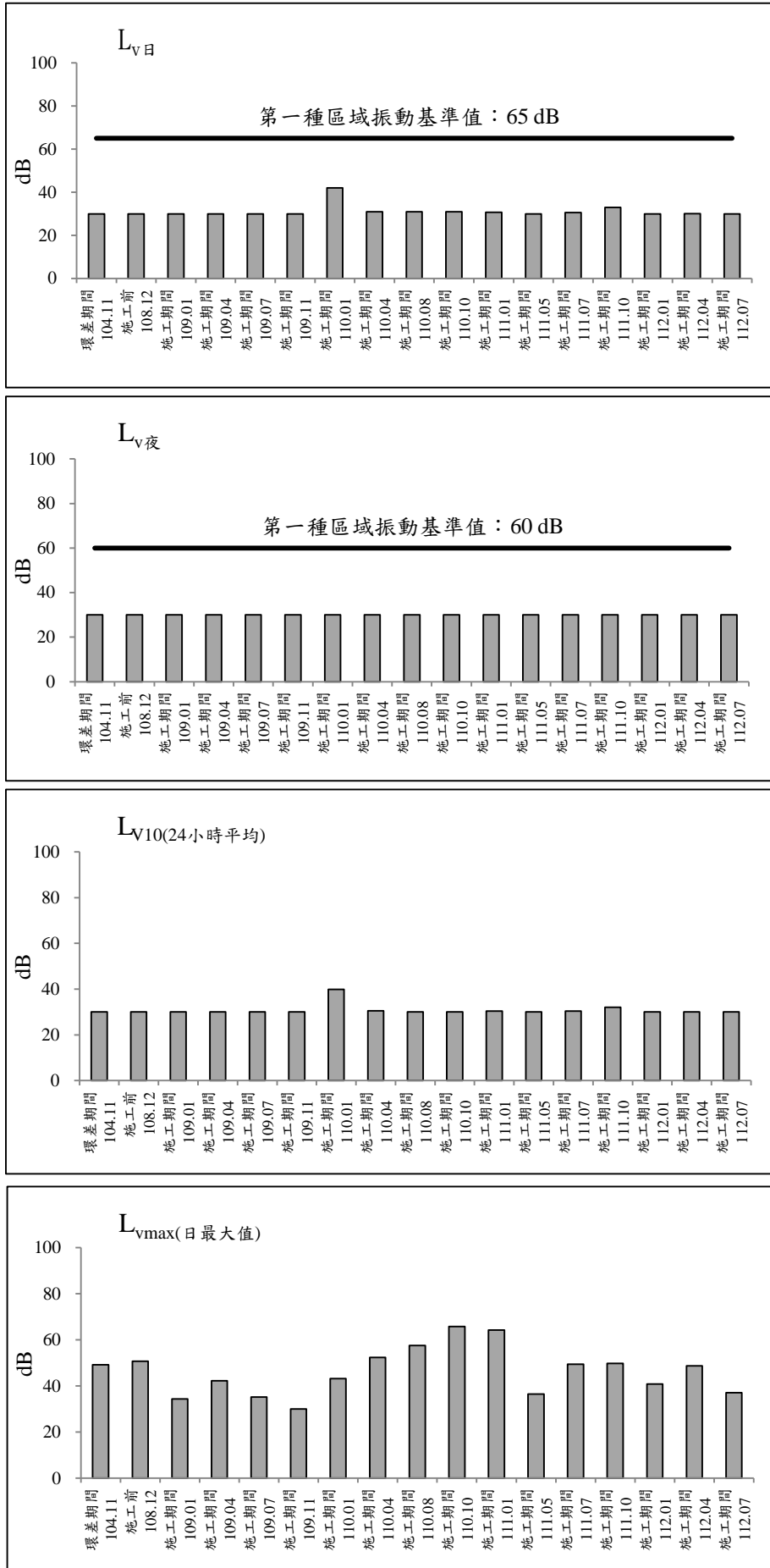
圖 2.2-10 鴻喜鎮社區測站歷次振動監測之各項測值變化圖(平日)
