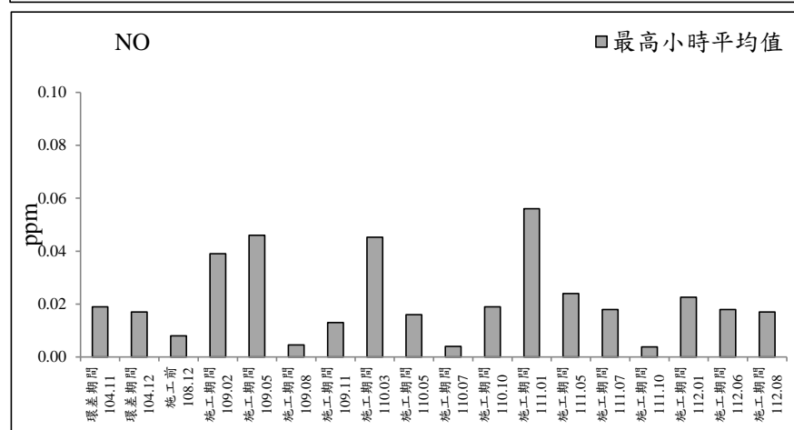
圖 2.1-1 鴻喜鎮社區測站歷次空氣品質監測之各項測值變化圖(續 1)
