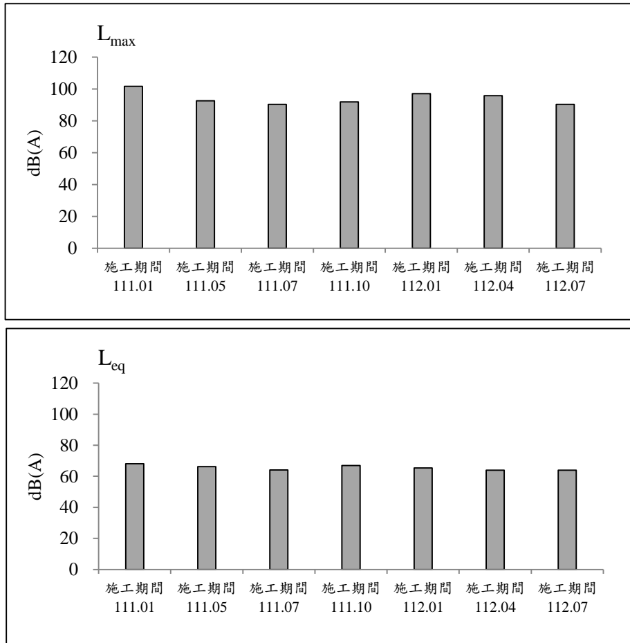
圖 2.2-8 保留戶(南興路二段230號民宅)測站歷次噪音監測之各項測值變化圖(平日)
