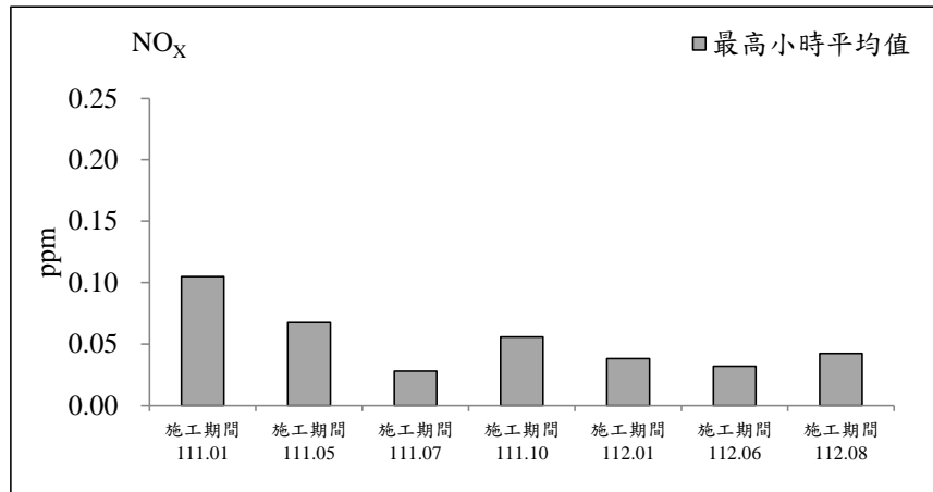
圖 2.1-4 保留戶(南興路二段 230 號民宅)測站歷次空氣品質監測之各項測值變化圖
