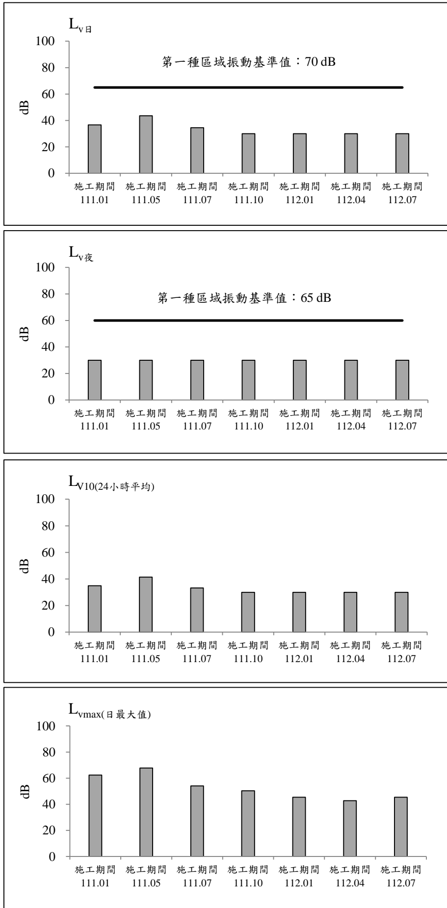
圖 2.2-16 保留戶(南興路二段230號民宅)測站歷次振動監測之各項測值變化圖(平日)
