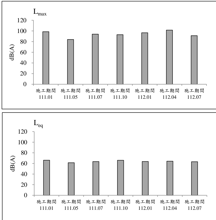
圖 2.2-7 保留戶(南興路二段230號民宅)測站歷次噪音監測之各項測值變化圖(假日)
