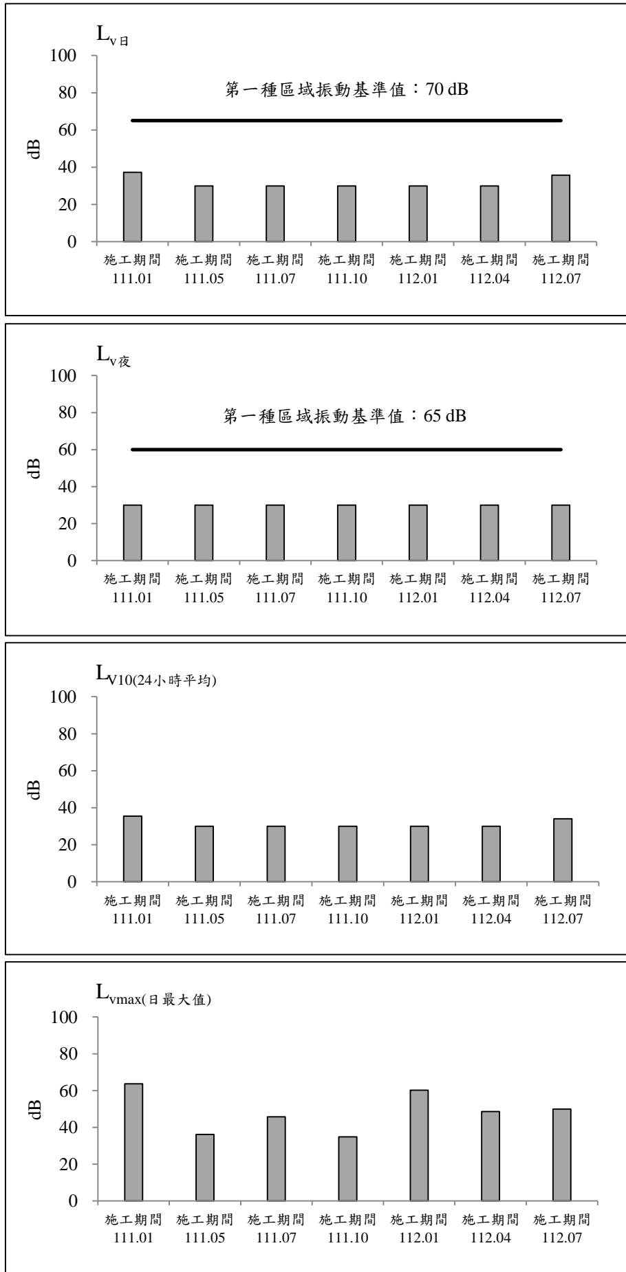
圖 2.2-15 保留戶(南興路二段230號民宅)測站歷次振動監測之各項測值變化圖(假日)
