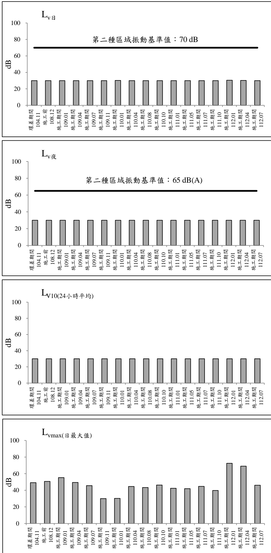
圖 2.2-12 台66線與縣112甲線交會口測站歷次振動監測之各項測值變化圖(平日)
