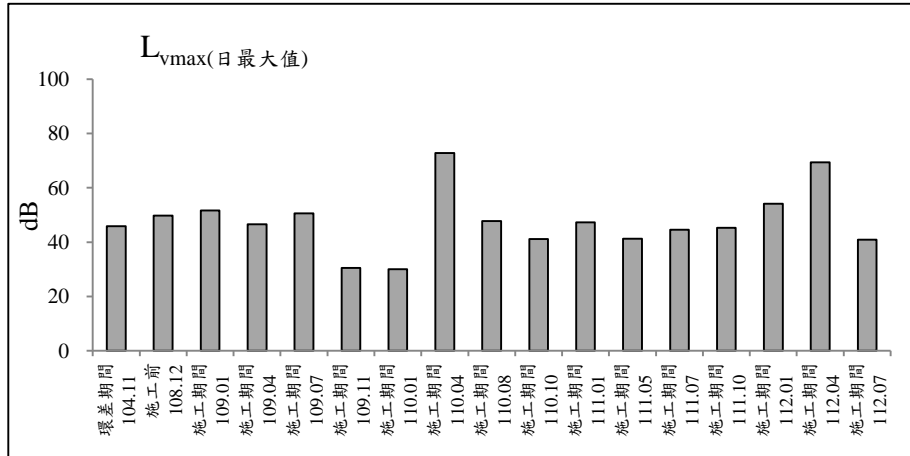
圖 2.2-11 台66線與縣112甲線交會口測站歷次振動監測之各項測值變化圖(假日)
