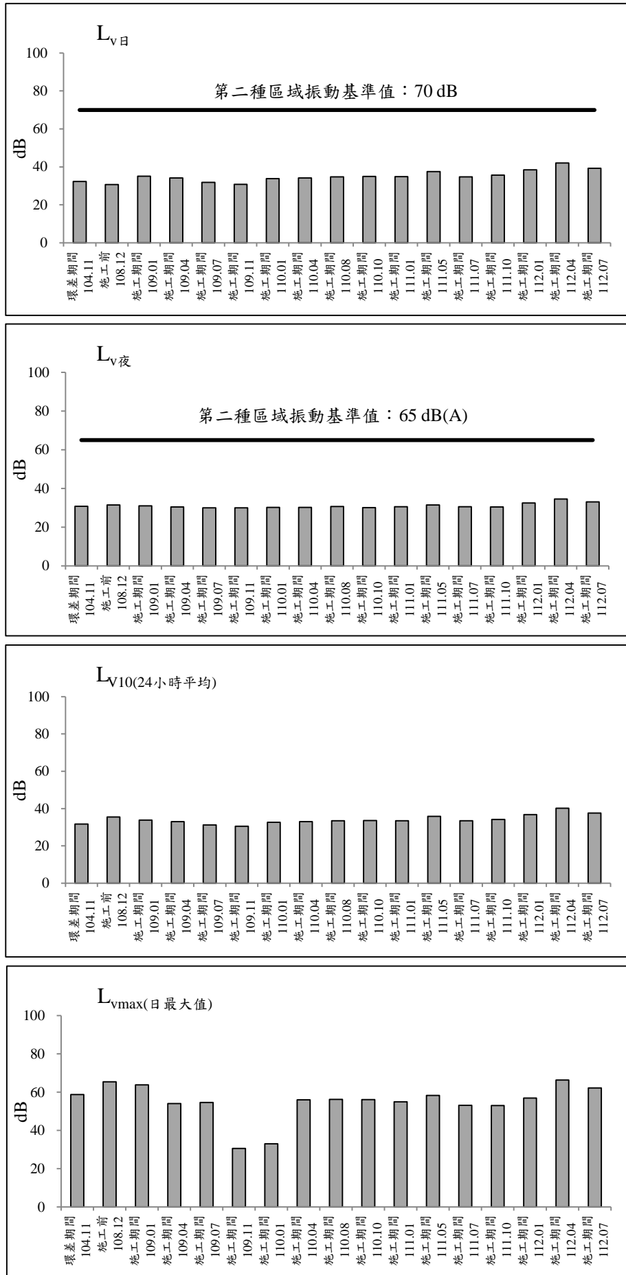
圖 2.2-14 縣112線與縣112甲線交會口測站歷次振動監測之各項測值變化圖(平日)
