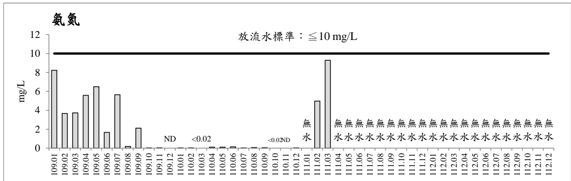
圖 2.7-2 歷次第二工區放流水監測之各項測值變化圖(續)
