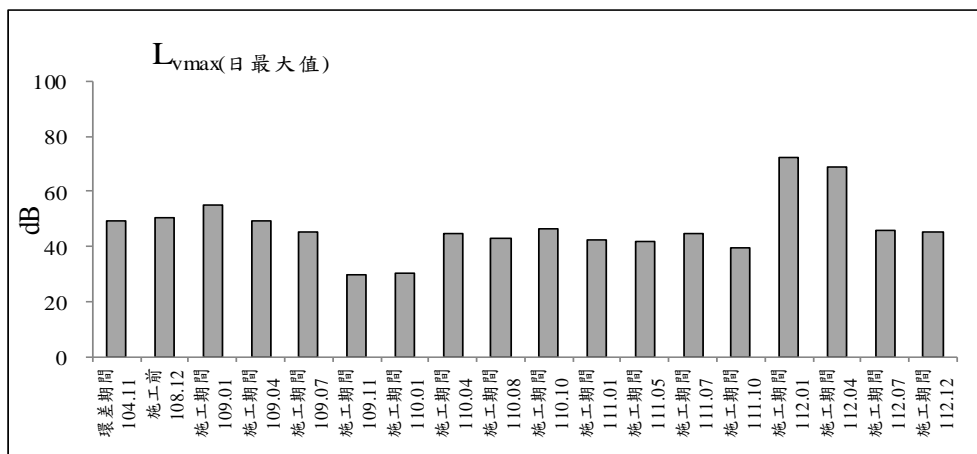
圖 2.2-12 台66線與縣112甲線交會口測站歷次振動監測之各項測值變化圖(平日)
