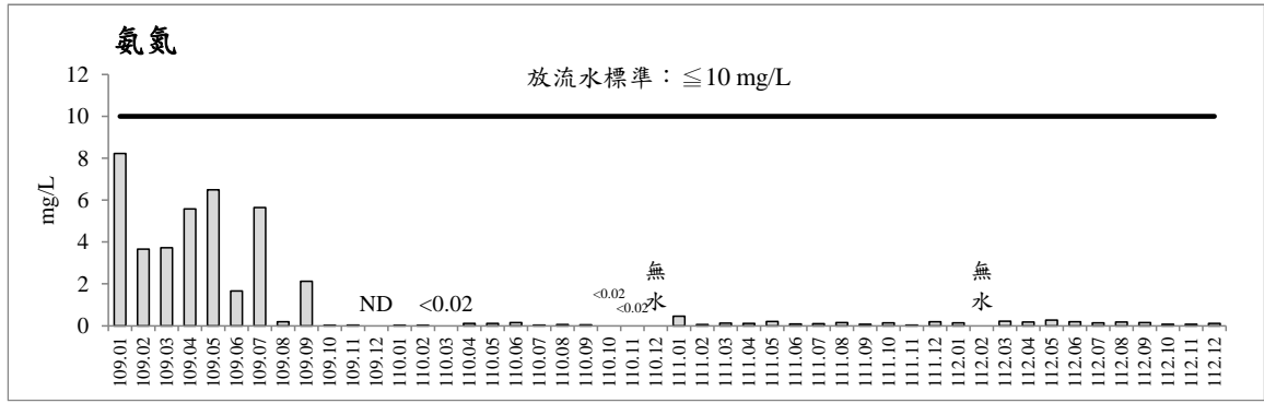
圖 2.7-4 歷次第四工區放流水監測之各項測值變化圖(續)
