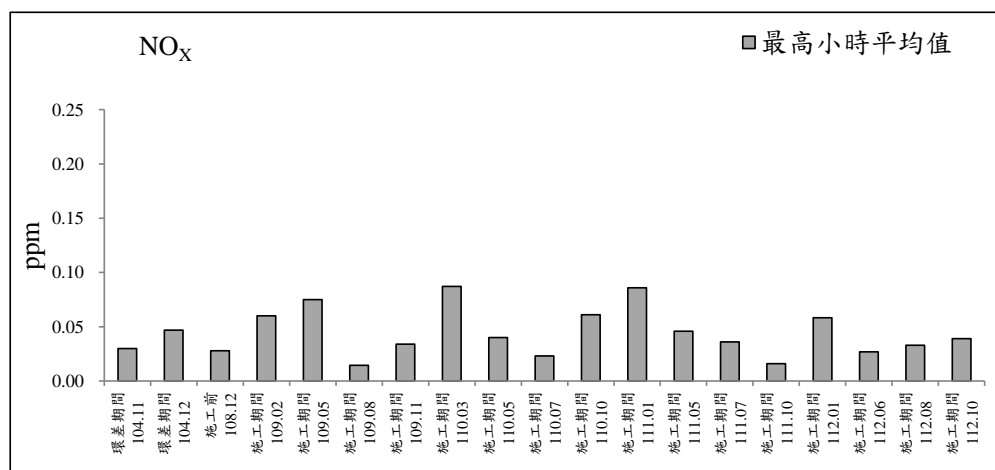
圖 2.1-1 鴻喜鎮社區測站歷次空氣品質監測之各項測值變化圖
