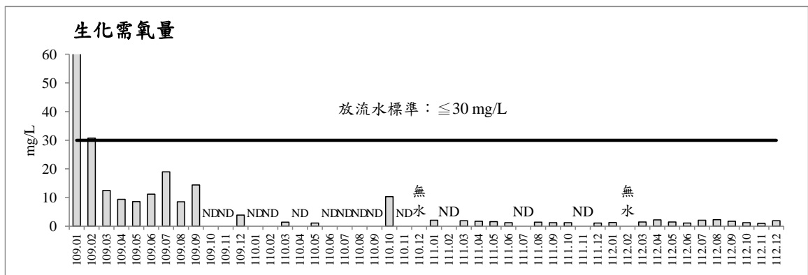
圖 2.7-4 歷次第四工區放流水監測之各項測值變化圖
