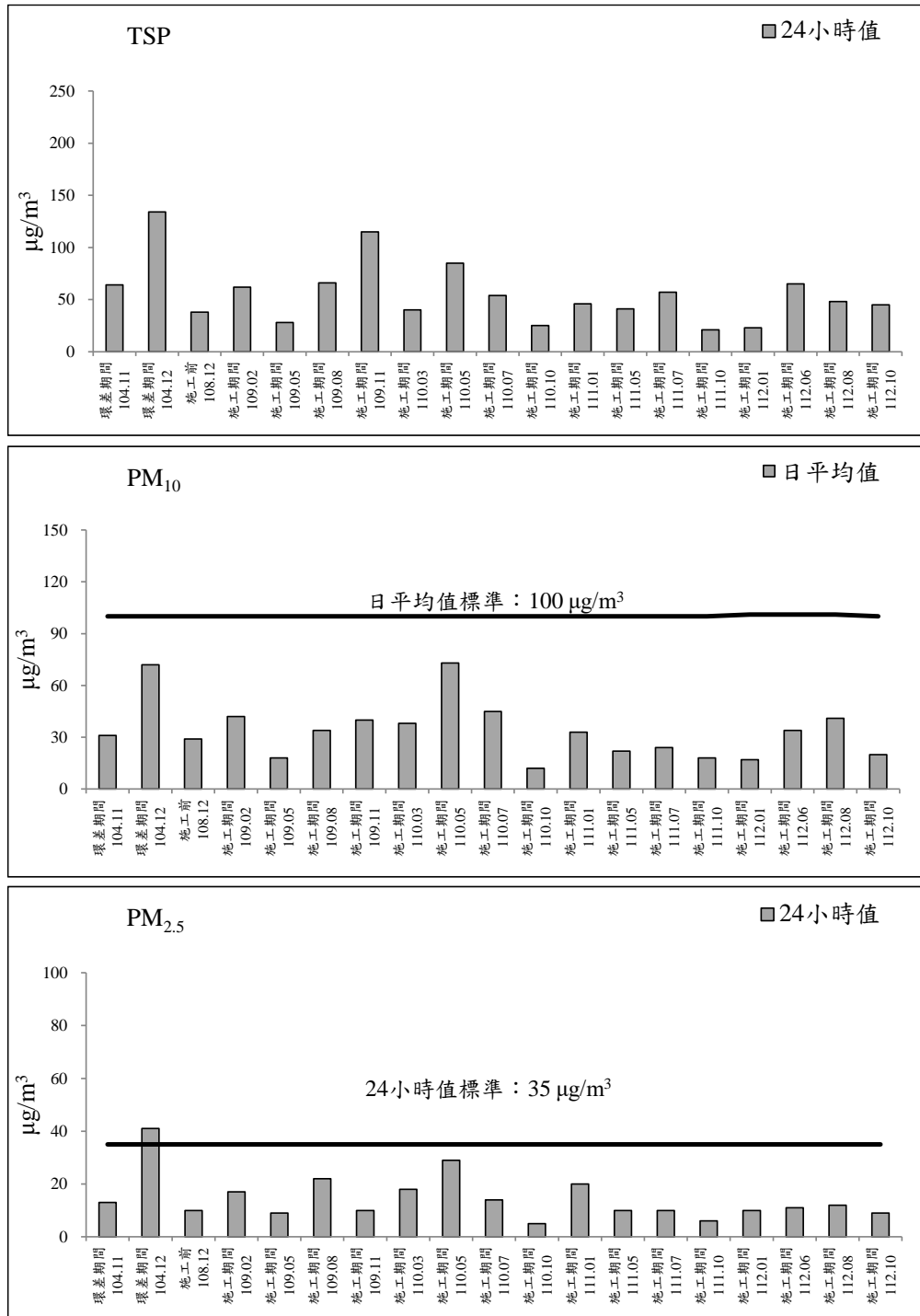
圖 2.1-2 永昌宮測站歷次空氣品質監測之各項測值變化圖(續 3)
