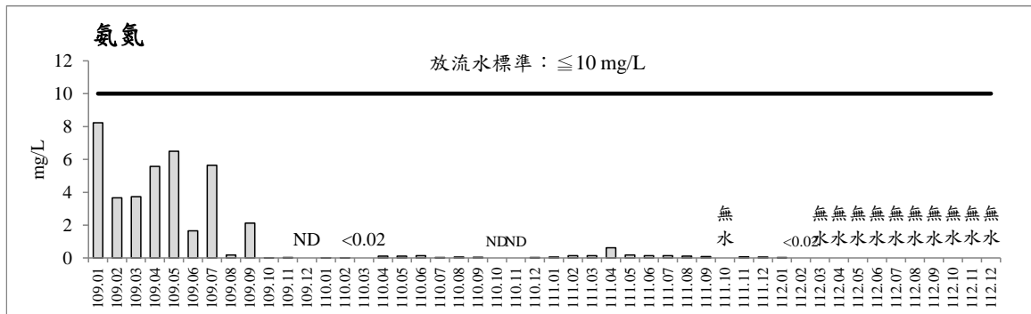
圖 2.7-1 歷次第一工區放流水監測之各項測值變化圖(續)
