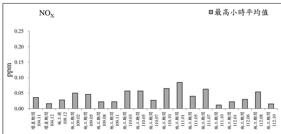
圖 2.1-2 永昌宮測站歷次空氣品質監測之各項測值變化圖
