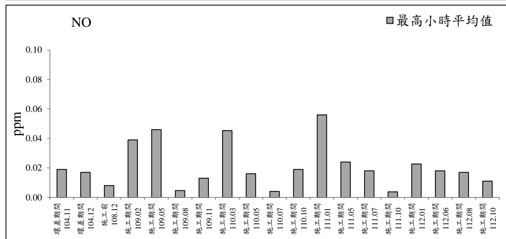
圖 2.1-1 鴻喜鎮社區測站歷次空氣品質監測之各項測值變化圖(續 1)
