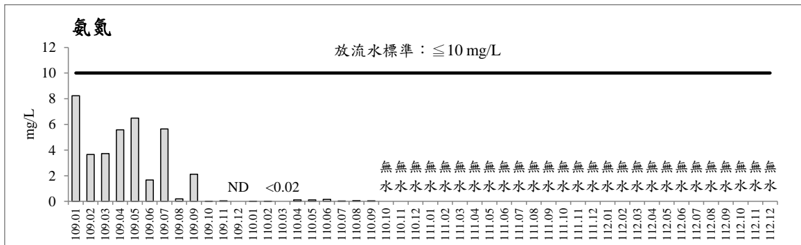
圖 2.7-3 歷次第三工區放流水監測之各項測值變化圖(續)
