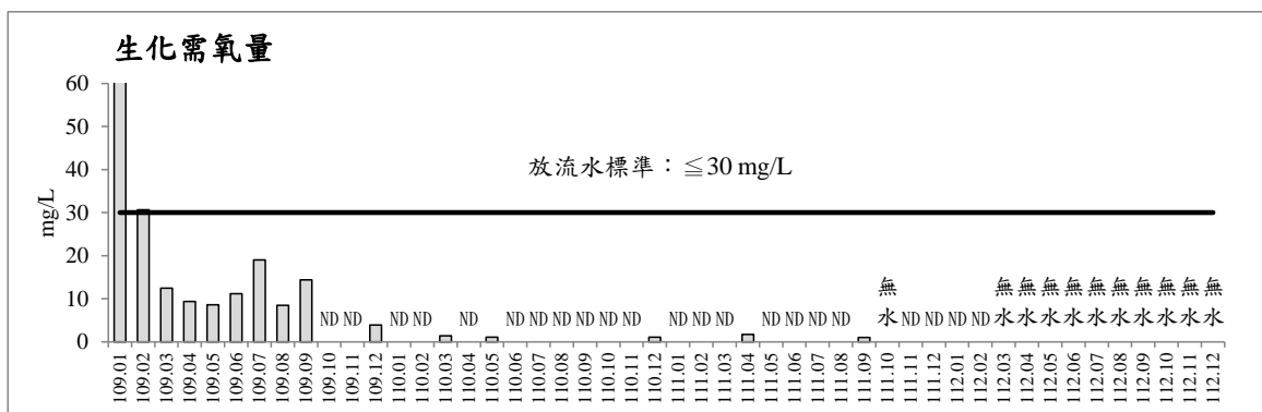
圖 2.7-1 歷次第一工區放流水監測之各項測值變化圖
