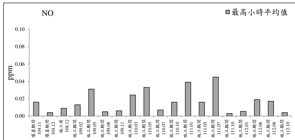
圖 2.1-2 永昌宮測站歷次空氣品質監測之各項測值變化圖(續 1)
