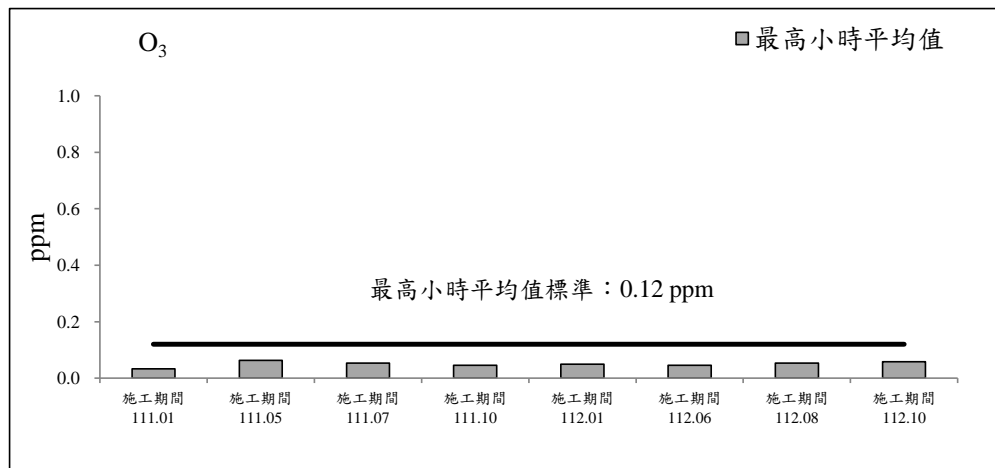
圖 2.1-2 永昌宮測站歷次空氣品質監測之各項測值變化圖(續 2)
