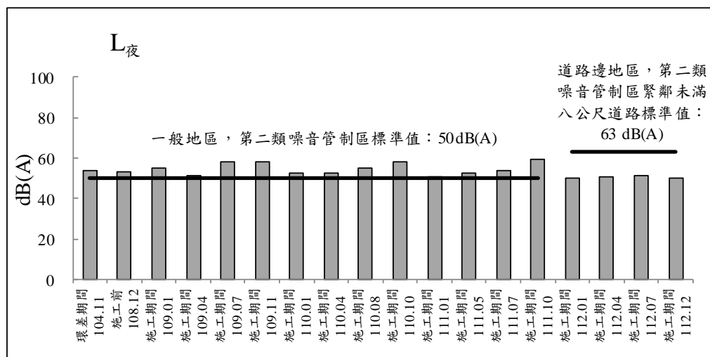
圖 2.2-2 鴻喜鎮社區測站歷次噪音監測之各項測值變化圖(平日)
