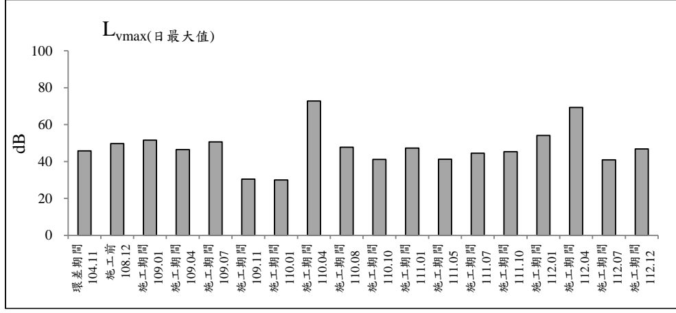
圖 2.2-11 台66線與縣112甲線交會口測站歷次振動監測之各項測值變化圖(假日)
