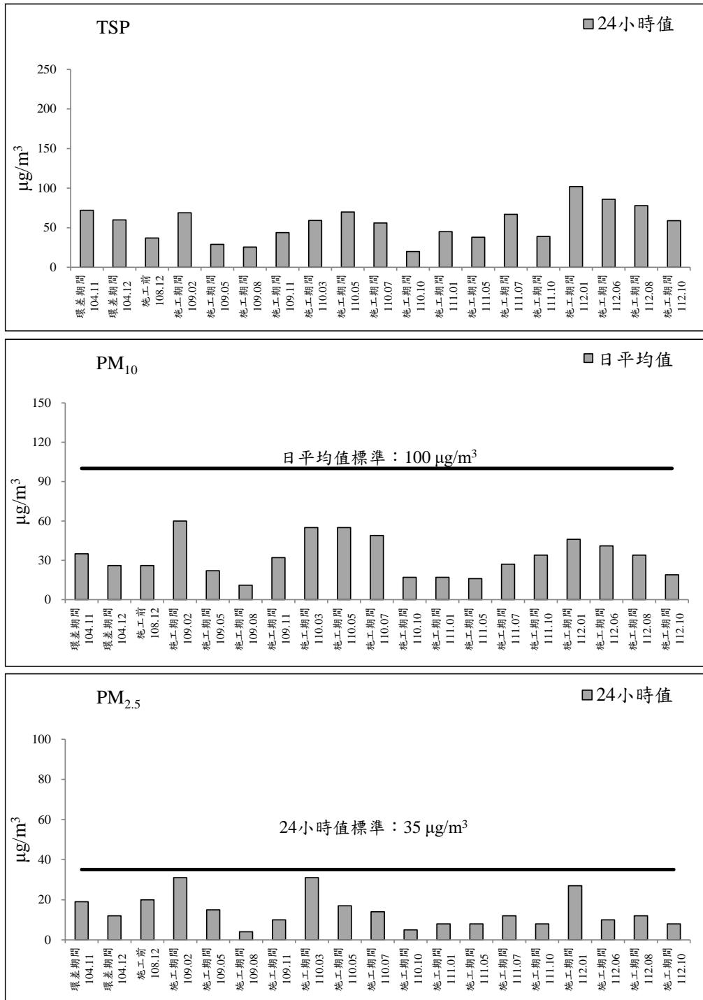
圖 2.1-1 鴻喜鎮社區測站歷次空氣品質監測之各項測值變化圖(續 3)
