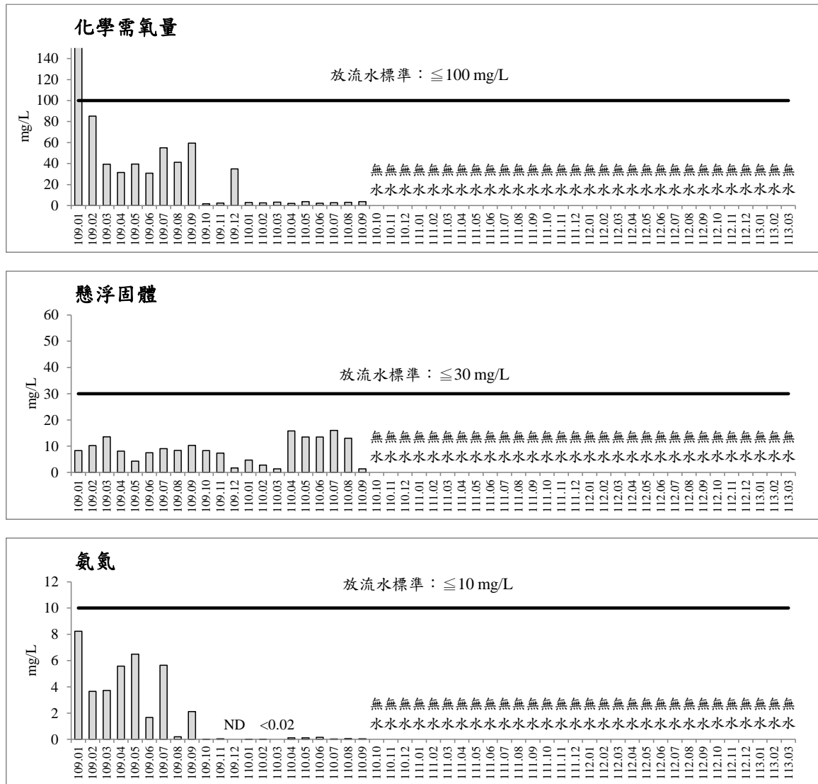
圖 2.7-3 歷次第三工區放流水監測之各項測值變化圖(續)
