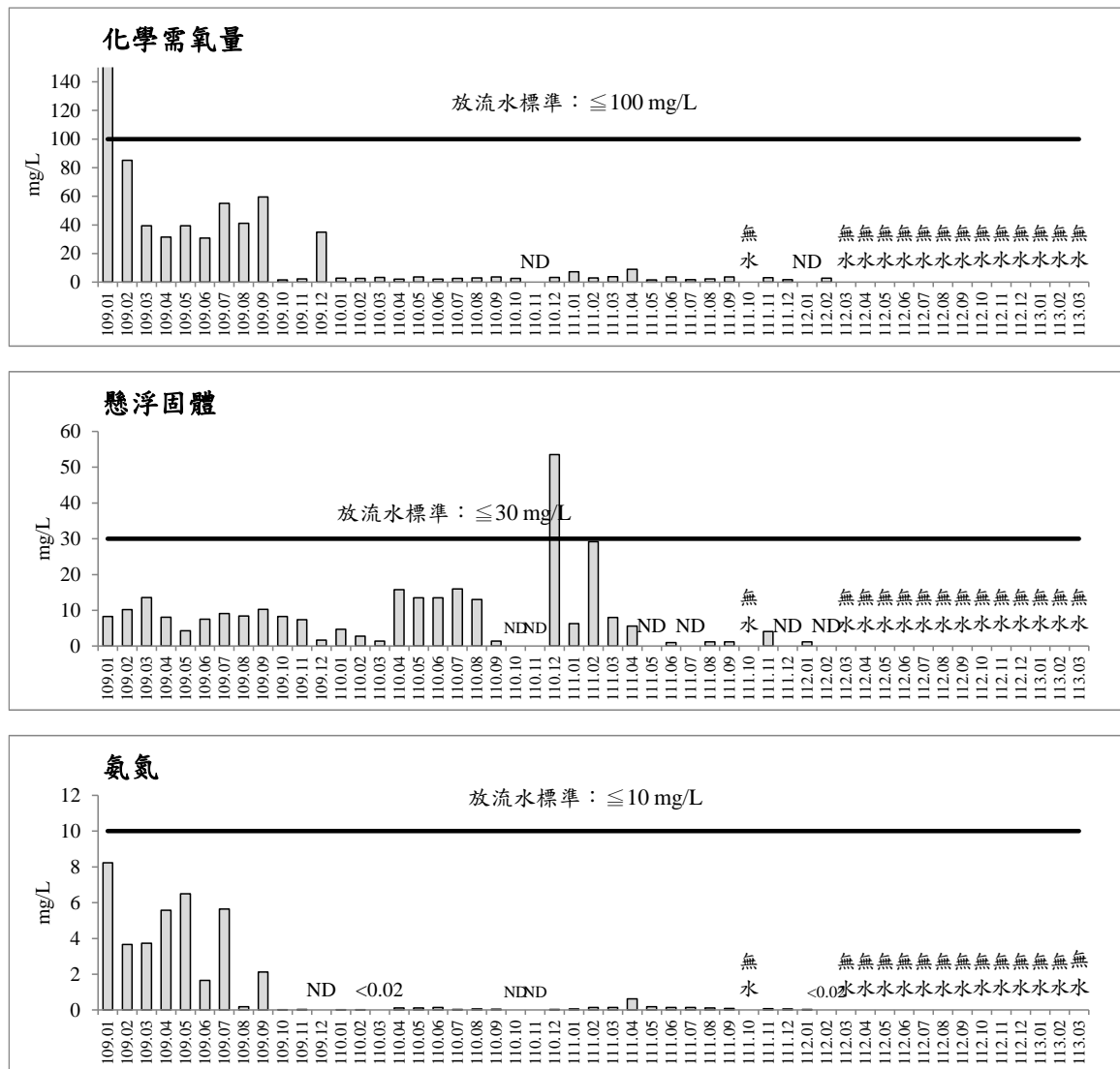
圖 2.7-1 歷次第一工區放流水監測之各項測值變化圖(續)
