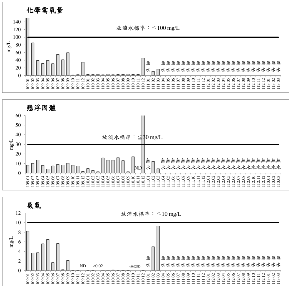
圖 2.7-2 歷次第二工區放流水監測之各項測值變化圖(續)
