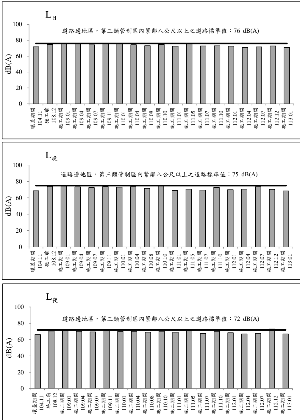
圖 2.2-3 台66線與縣112甲線交會口測站歷次噪音監測之各項測值變化圖(假日)
