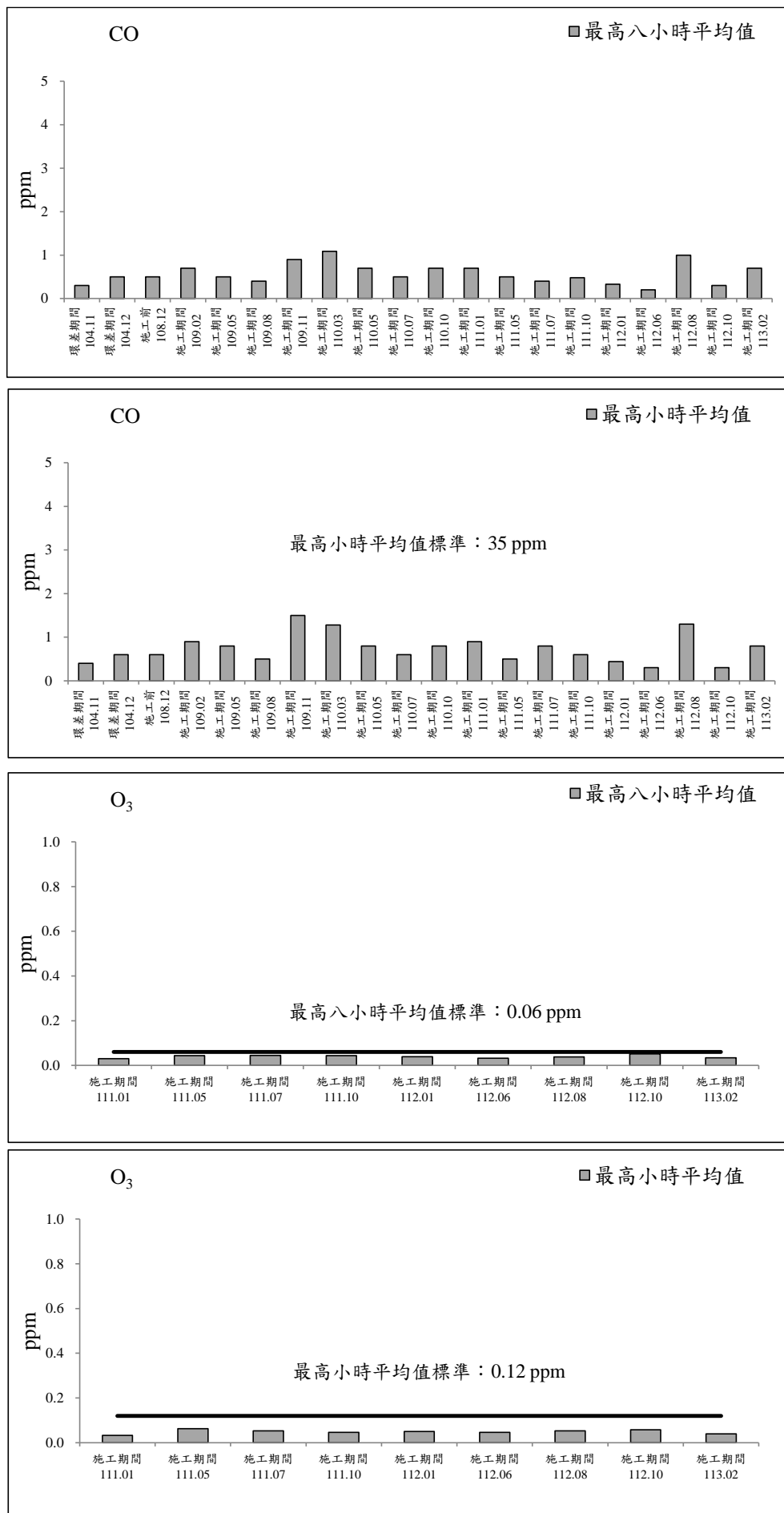
圖 2.1-2 永昌宮測站歷次空氣品質監測之各項測值變化圖(續 2)
