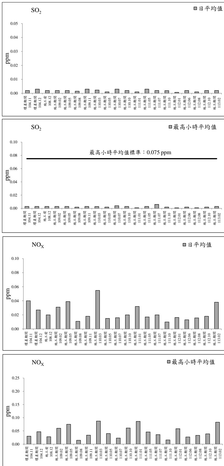
圖 2.1-1 鴻喜鎮社區測站歷次空氣品質監測之各項測值變化圖
