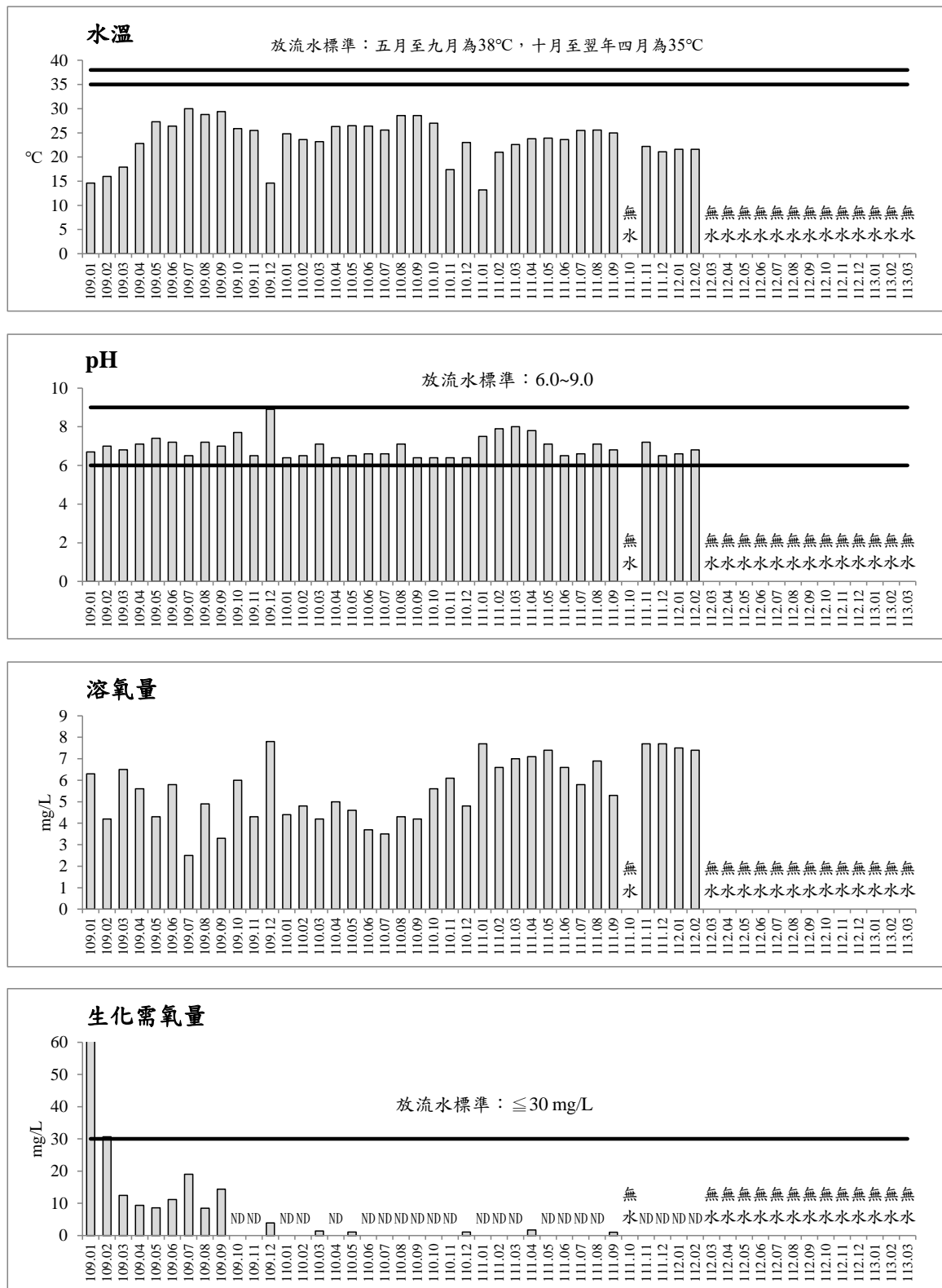
圖 2.7-1 歷次第一工區放流水監測之各項測值變化圖
