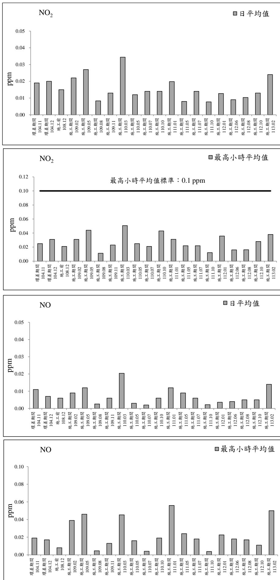
圖 2.1-1 鴻喜鎮社區測站歷次空氣品質監測之各項測值變化圖(續 1)
