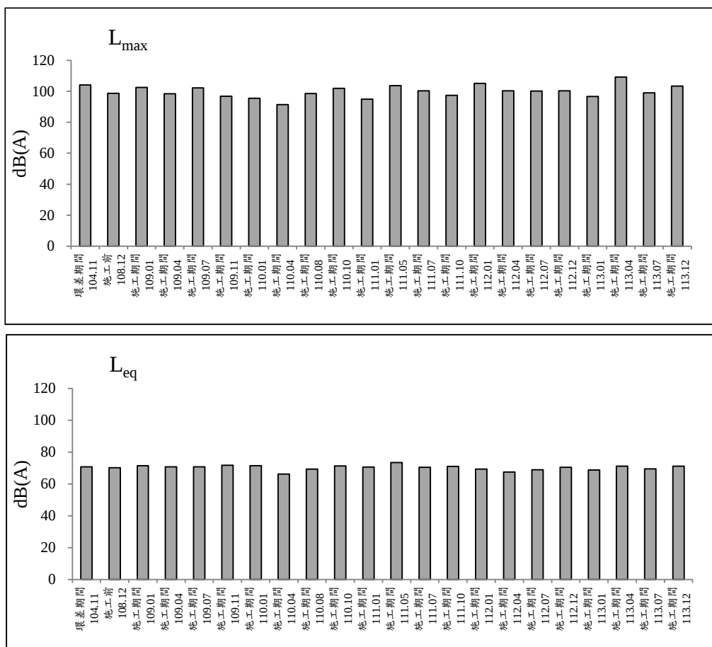
圖 2.2-5 縣112線與縣112甲線交會口測站歷次噪音監測之各項測值變化圖(假日)(續)
