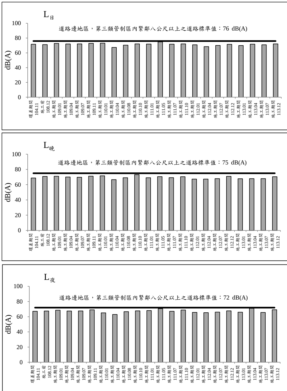
圖 2.2-5 縣112線與縣112甲線交會口測站歷次噪音監測之各項測值變化圖(假日)
