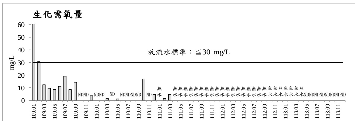
圖 2.7-2 歷次第二工區放流水監測之各項測值變化圖
