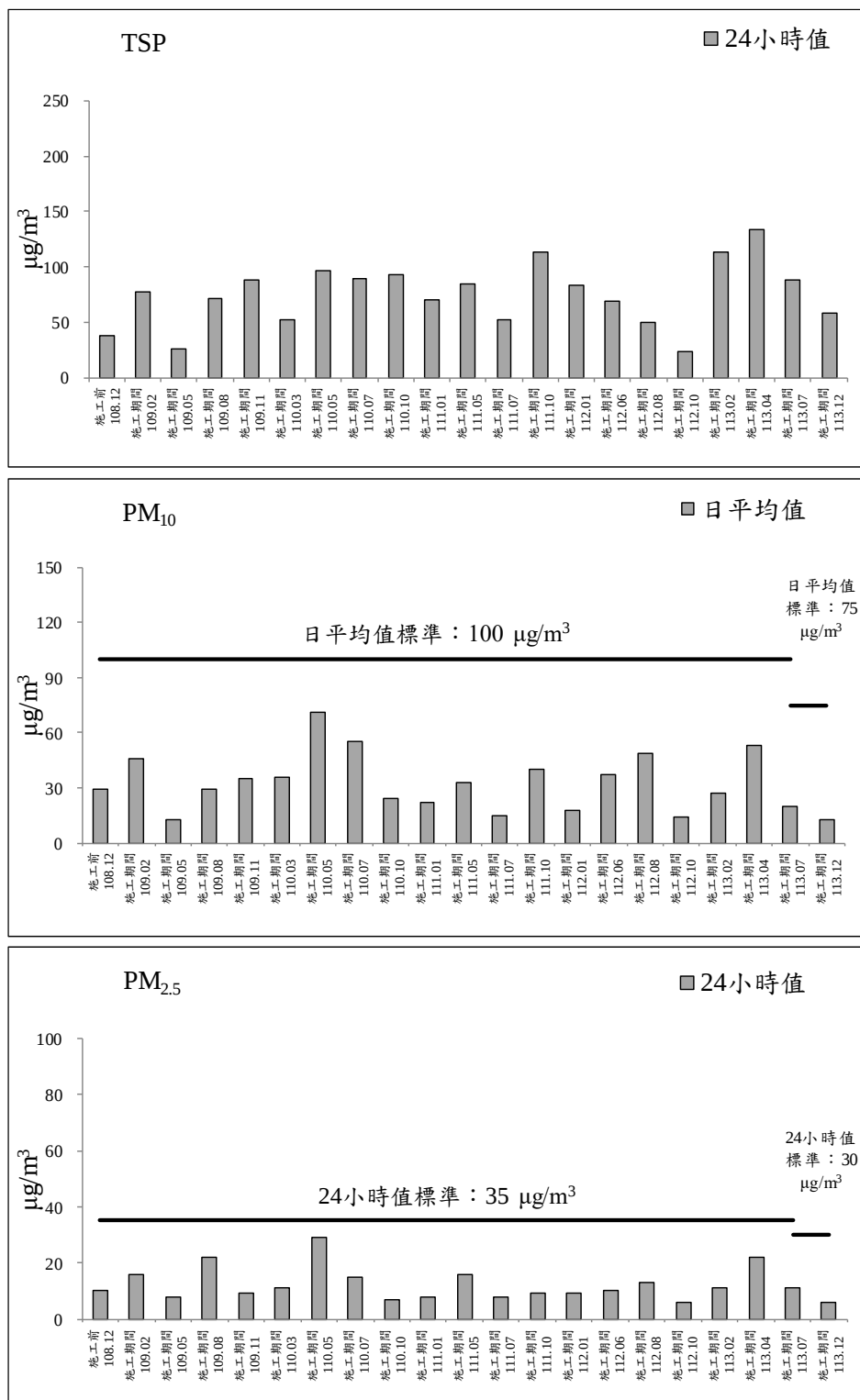
圖 2.1-3 南興路二段 52 巷測站歷次空氣品質監測之各項測值變化圖 (續 3)
