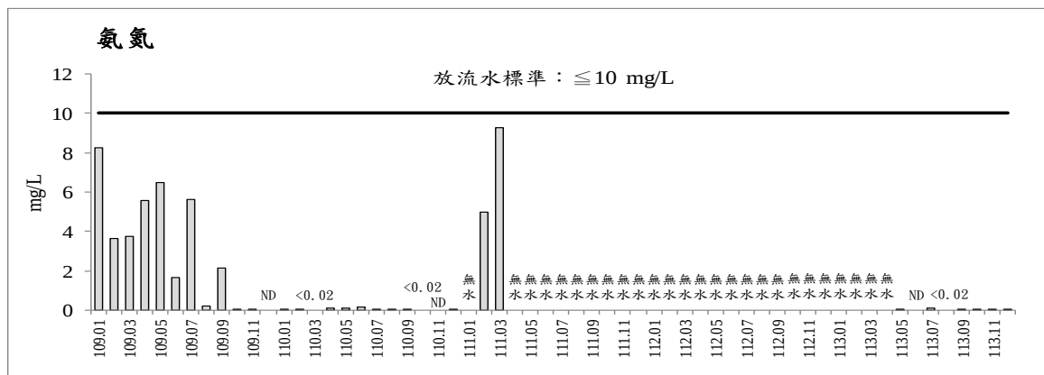
圖 2.7-2 歷次第二工區放流水監測之各項測值變化圖(續)
