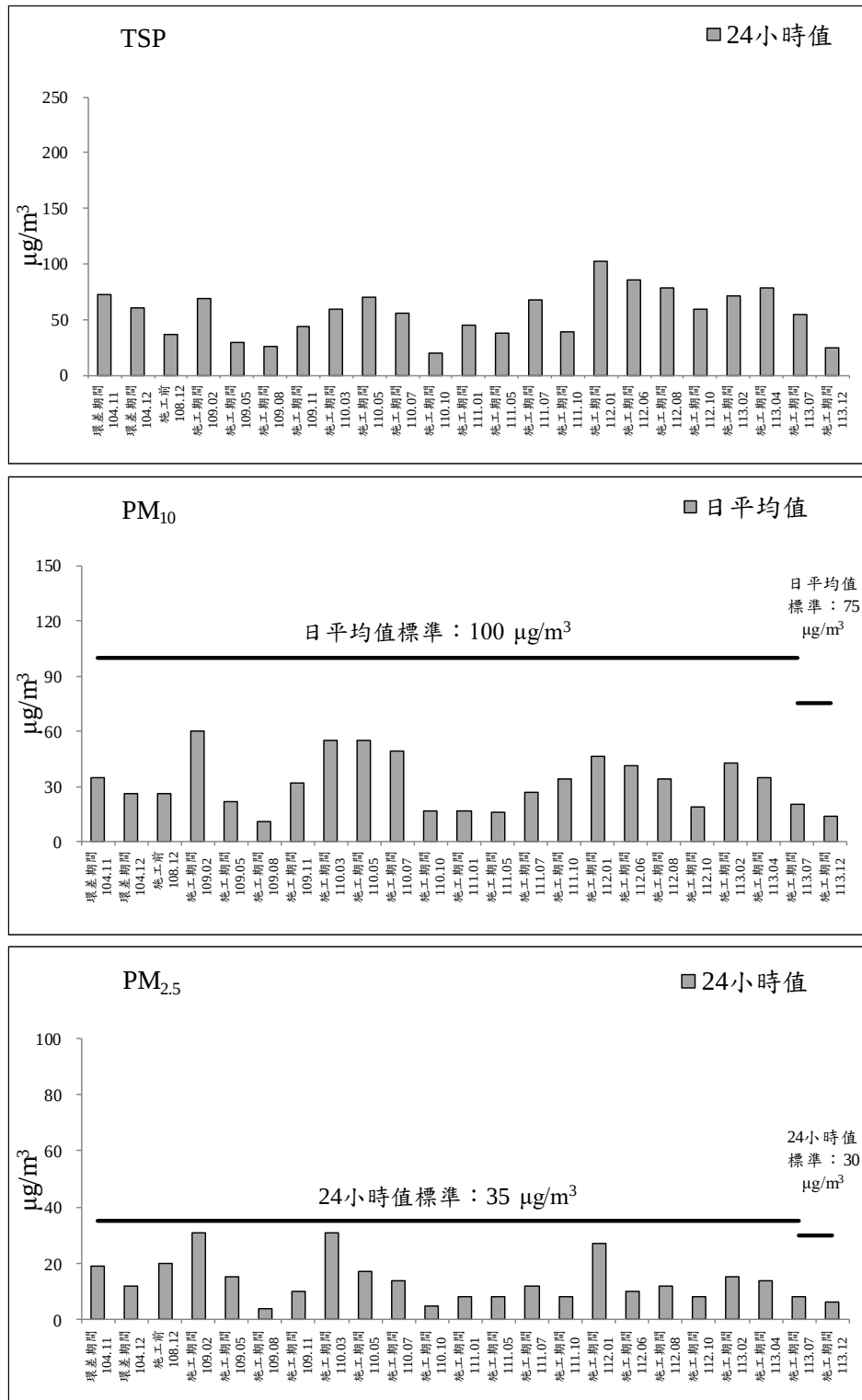
圖 2.1-1 鴻喜鎮社區測站歷次空氣品質監測之各項測值變化圖(續 3)
