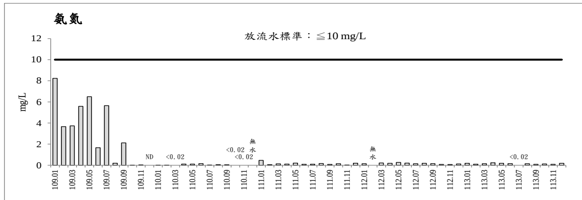
圖 2.7-4 歷次第四工區放流水監測之各項測值變化圖(續)
