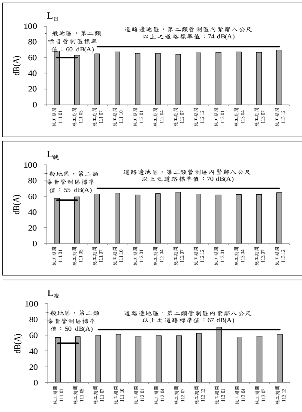
圖 2.2-7 保留戶(南興路二段230號民宅)測站歷次噪音監測之各項測值變化圖(假日)
