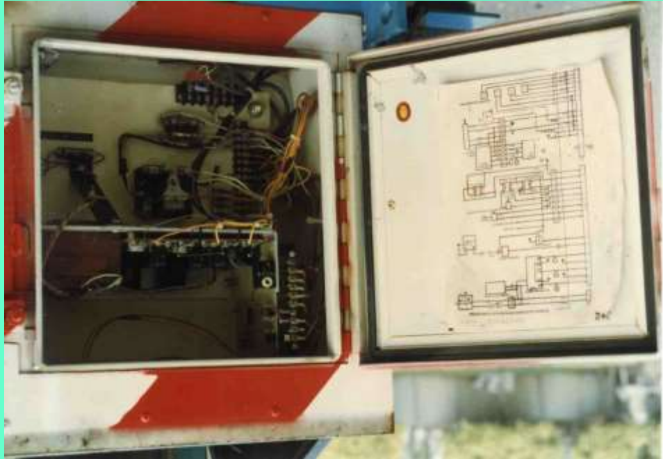
ROAD RATER 電路系統
