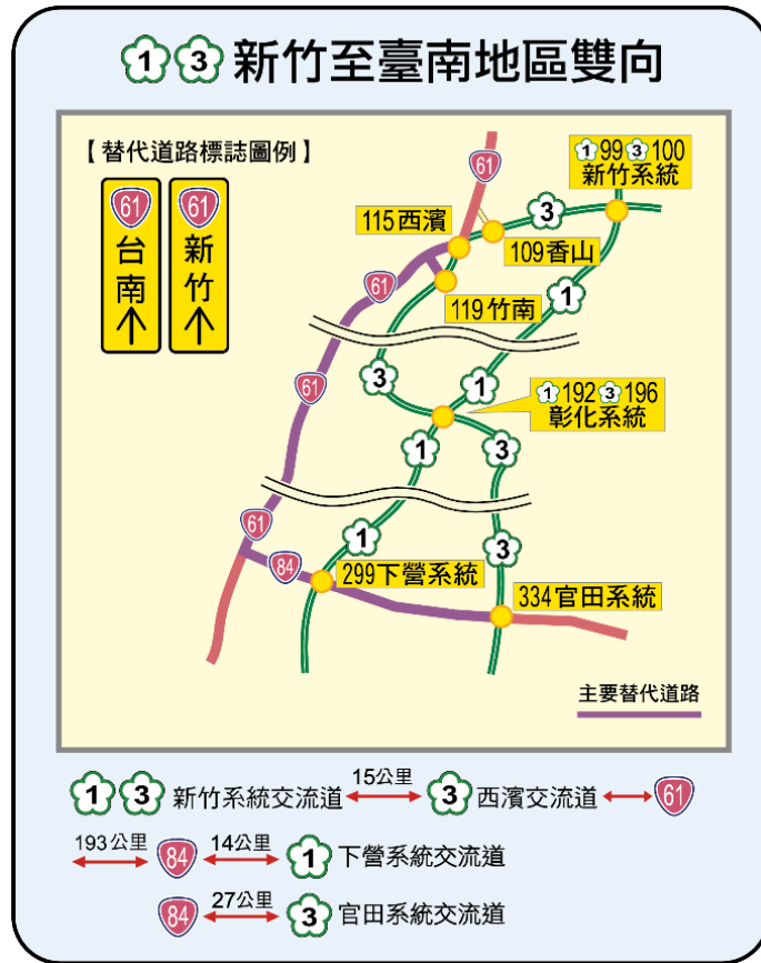
附圖 3 國 1 國 3 新竹-臺南地區雙向替代道路圖
